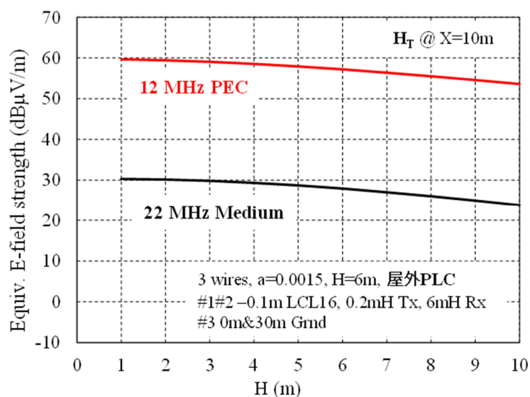
図 5.25 離隔距離 10m における磁界強度（等価電界強度）： 金属大地(PEC)と一般土壌(Medium)との比較
