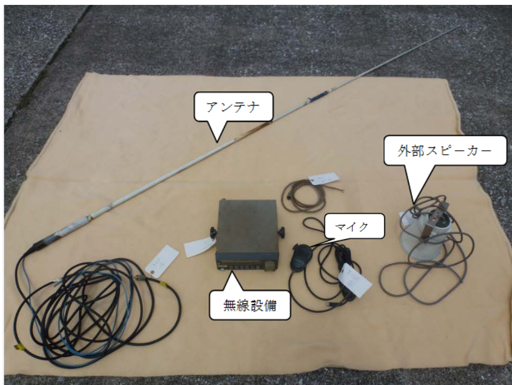
<船舶に設置されていた不法無線設備>
