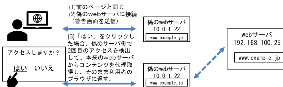
【図3 DNS+プロキシ方式②】 22
