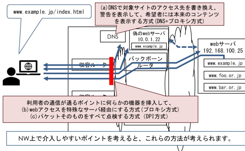
【図1 アクセス警告方式の実装方法】 18
