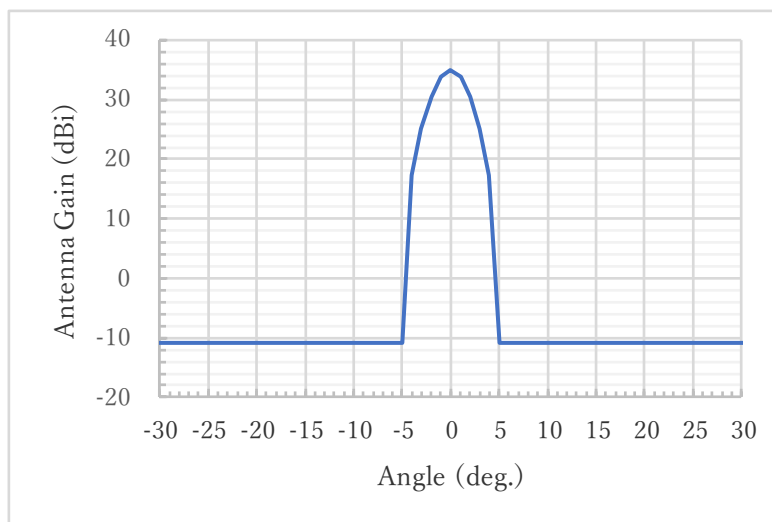
FPU のアンテナパターン (IEEE モデルによるシミュレーション)
