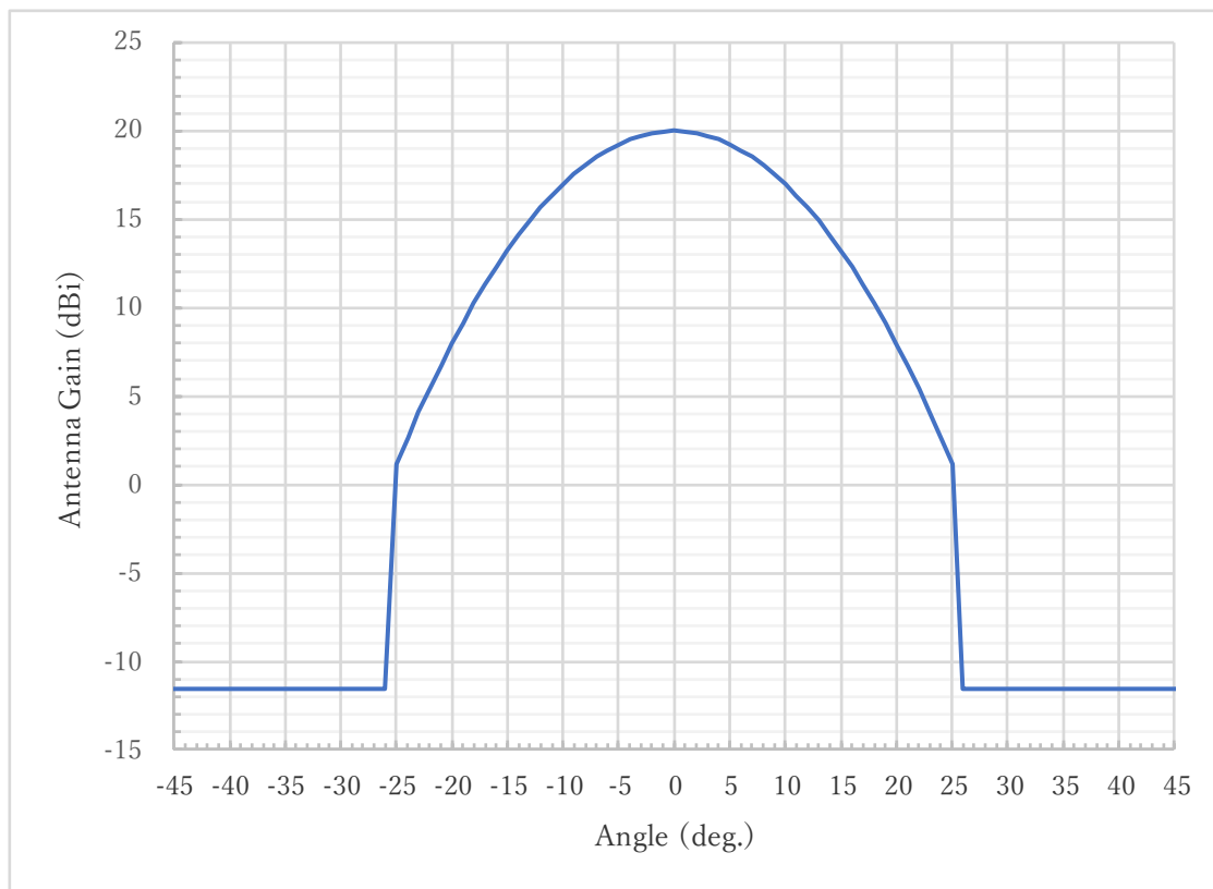
FWA システムのアンテナパターンシミュレーションの例 Beam= 20 [deg.], G= 20 [dBi], sidelobe= 26 [deg.], -11.55 [dBi]
