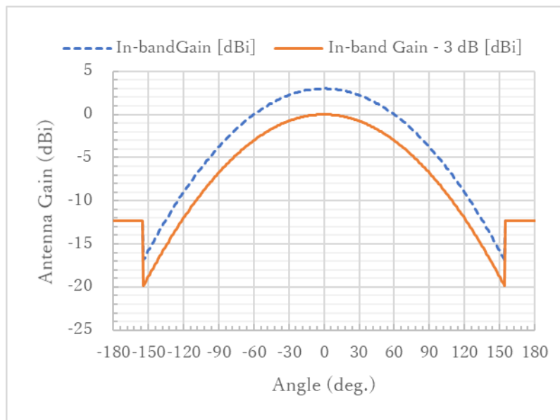
ミリ波センサーシステムのアンテナパターン (シミュレーション) Beam= 120 [deg.], G= 0 [dBi], Sidelob= 154 [deg.], -19.83 [dBi]
