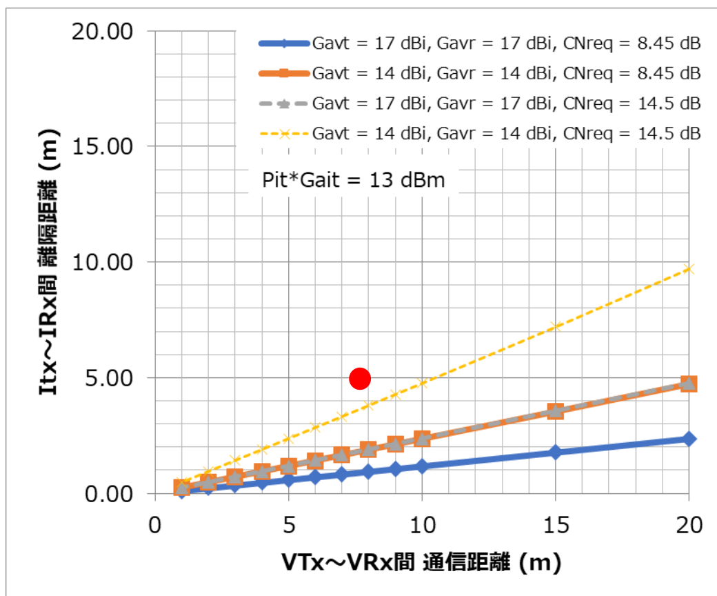
図 4-3-3 WiGigの通信距離に対する与干渉装置との所要離隔距離
