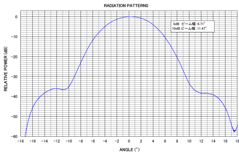
ミリ波画像伝送システムのアンテナパターン Beam= 6.71 [deg.], G= 23 [dBi]
