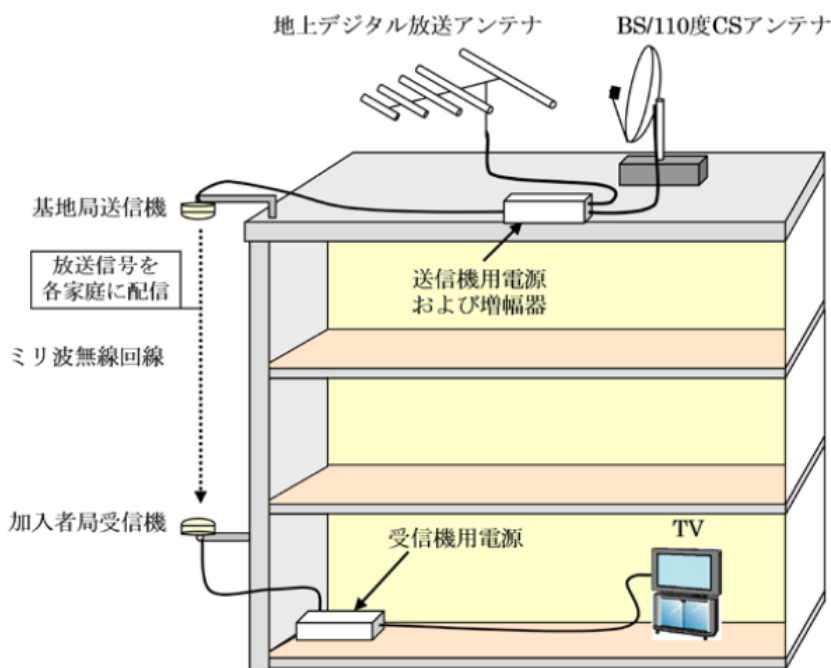
ミリ波画像伝送システムの代表的な運用形態
