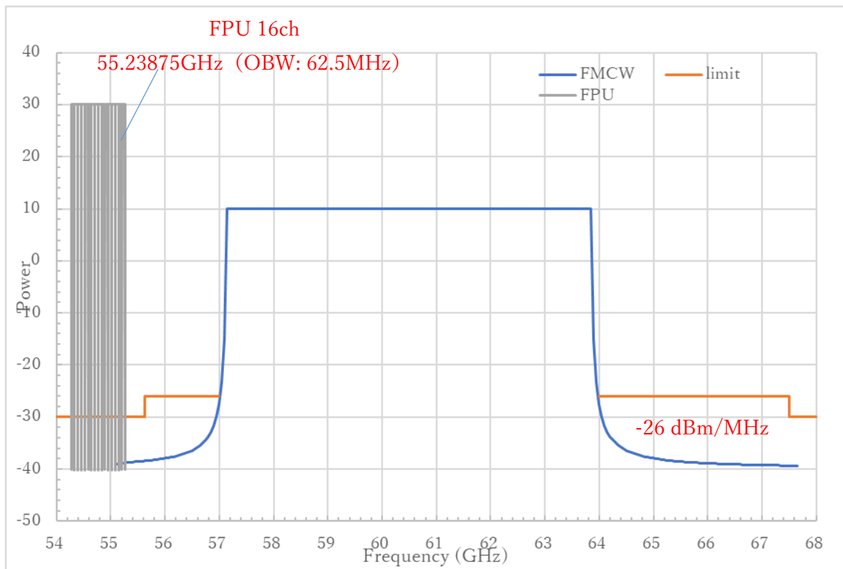
FPU とミリ波センサーシステムの周波数関係
