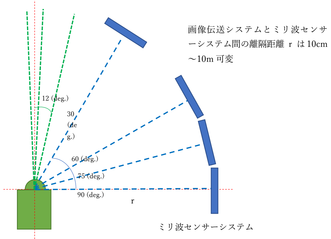
ミリ波画像伝送システムの受信機
