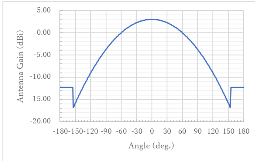
ミリ波センサーシステムのアンテナパターン (シミュレーション) Beam= 120 [deg.], G= 3 [dBi], Sidelob= 154 [deg.], -16.83 [dBi]
