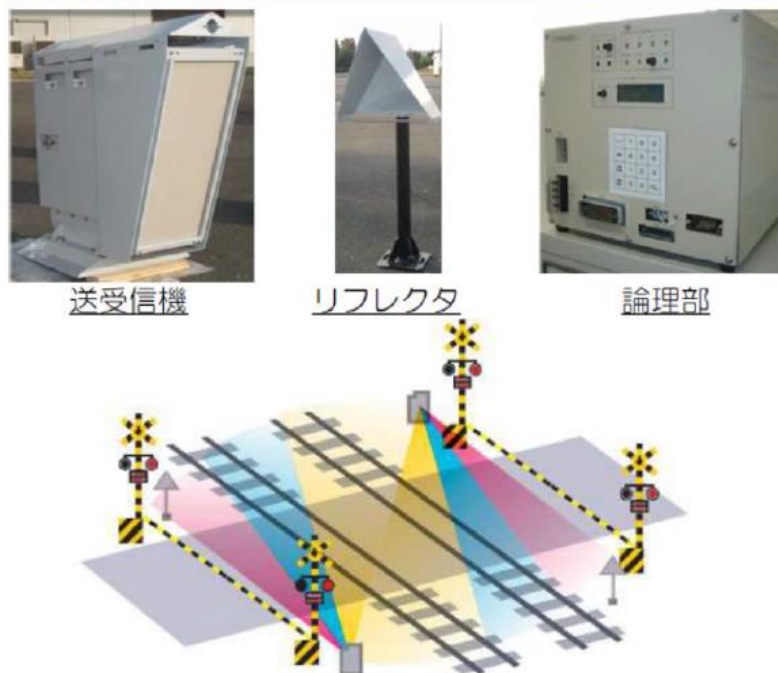
図 4-3-1 ミリ波踏切障害物検知装置
