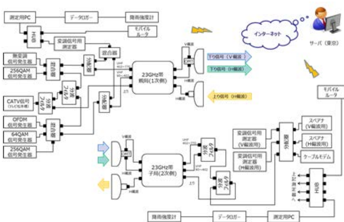
図 4-7 測定系統図
