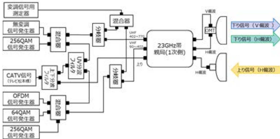
図 4-34 系統図 親局（1次）側
