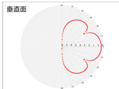
空中線指向特性
