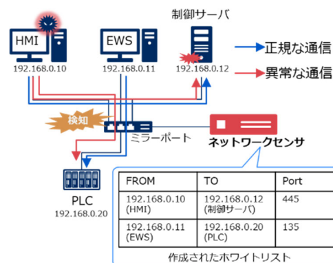
図3-3-2-3-2 ホワイトリスト方式の検知イメージ
