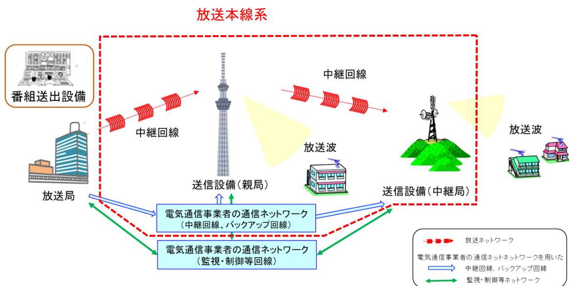
図 3-2-1 放送本線系（中継回線設備、放送局の送信設備）の構成例
