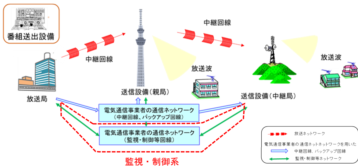
図 3-2-2 監視・制御設備系の構成例
