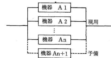
n + 1 予備方式
