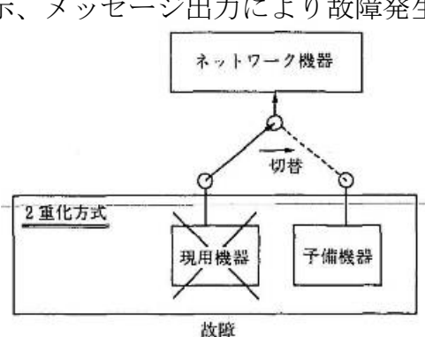
予備機器への切換え（2重化方式）
