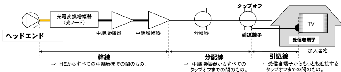
図2-2-3-2 HFC方式による設備の構成例
