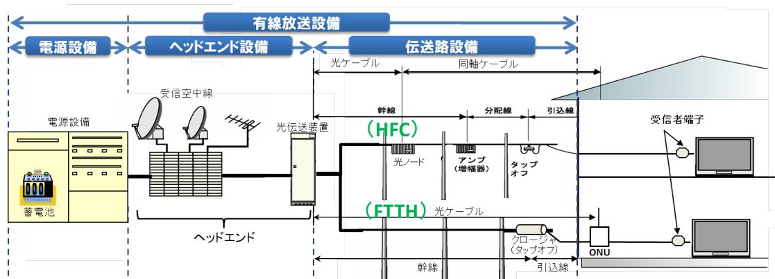
図2-2-3-1 有線放送に関する設備の構成例
