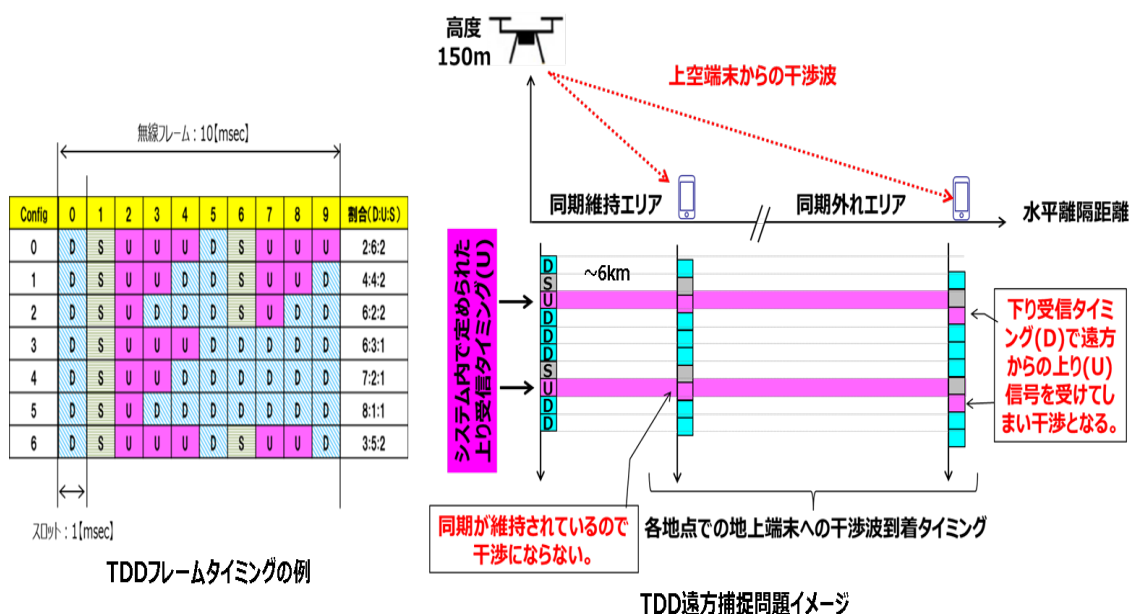
図 2. 2. 1 - 1 TDD 方式の遠方捕捉
