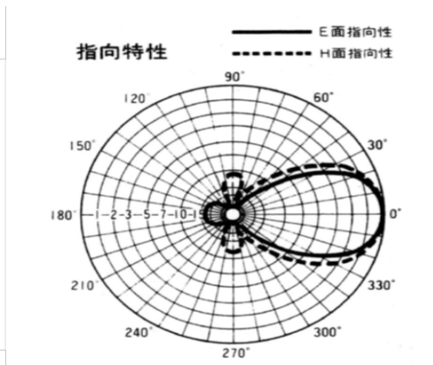
MCA水平、垂直面(管理移動) (P293 図. 添2-25)
