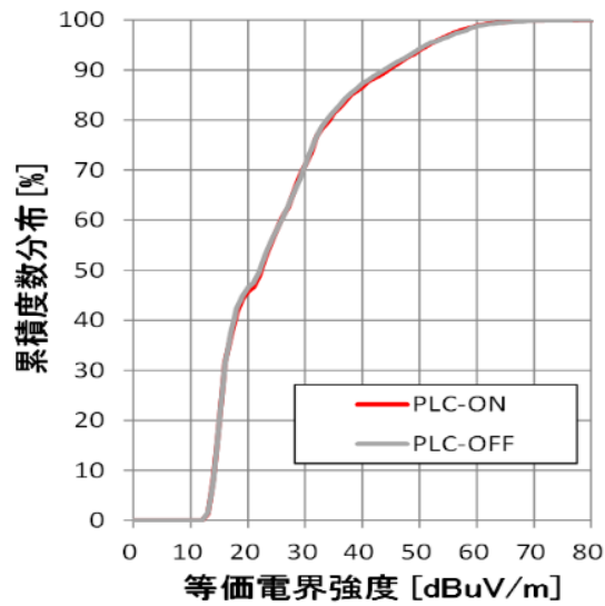
(b) PLC 設備の ON/OFF 時における累積分布
