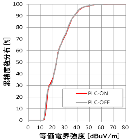
(b)PLC 設備 ON/OFF 時の磁界強度の累積分布
