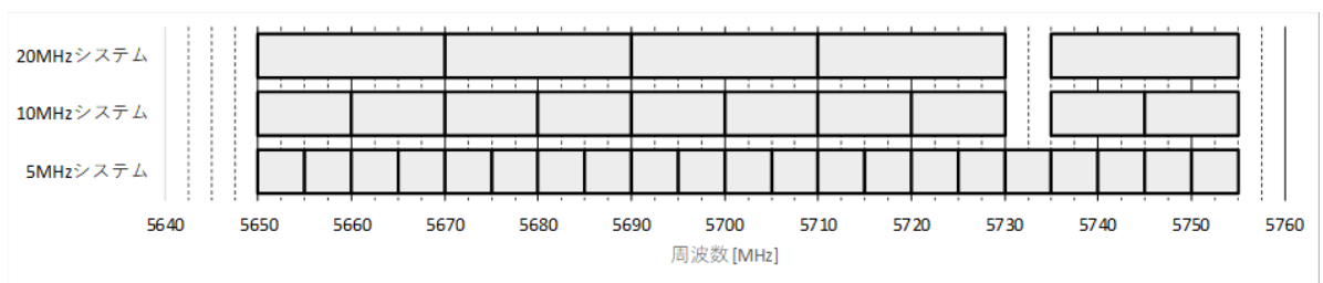
図 3.1.7 無人移動体画像伝送システムにおけるチャンネル配置
