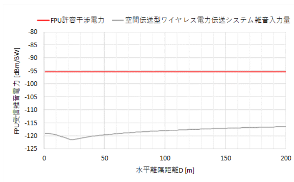
図参 6.4.3 水平離隔距離に対すると FPU システムに受信する空間伝送型ワイヤレス電力伝送システム雑音電力の関係
