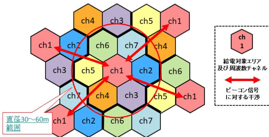
システム及び周波数チャンネル配置
