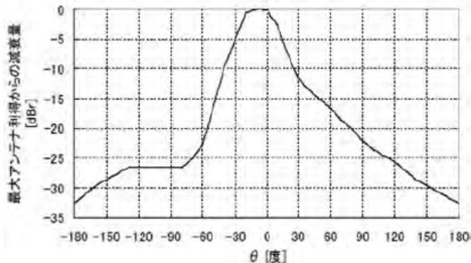
図参 1. 2. 1 垂直面内指向特性
