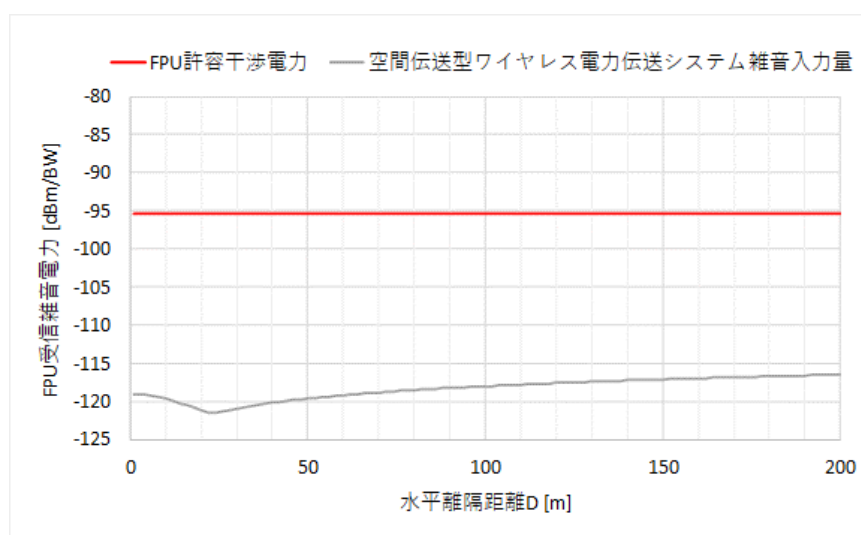
図 3.3.19 水平離隔距離に対すると FPU システムに受信する空間伝送型ワイヤレス電力伝送システム雑音電力の関係
