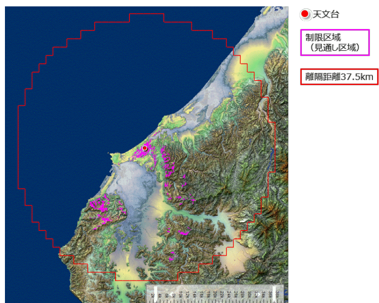
図参 4. 4. 7 あらわ観測所における空間伝送型ワイヤレス電力伝送システムの制限区域
