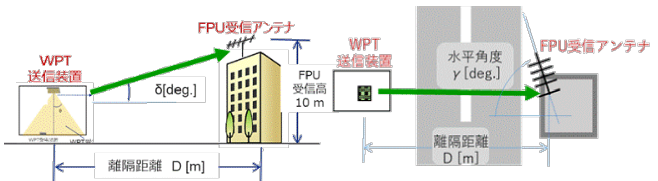
図 3.3.11 FPU ユースケースでの検討例
