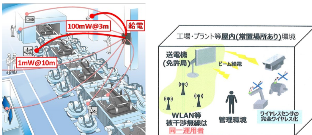
(a)工場内のセンサ
