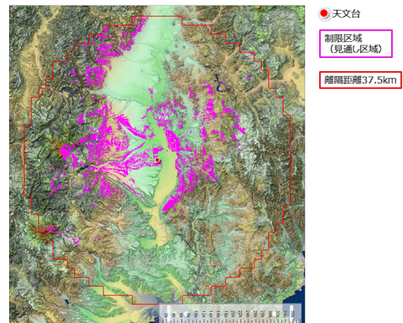
図 3. 3. 7 水沢観測所における空間伝送型ワイヤレス電力伝送システムの制限区域
