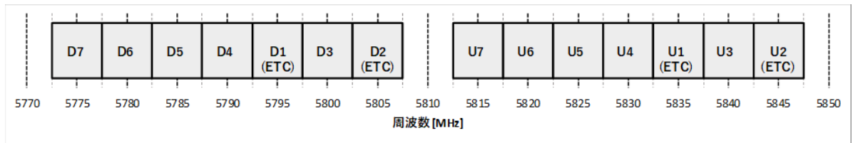
図 3.1.6 DSRC におけるチャンネル配置
