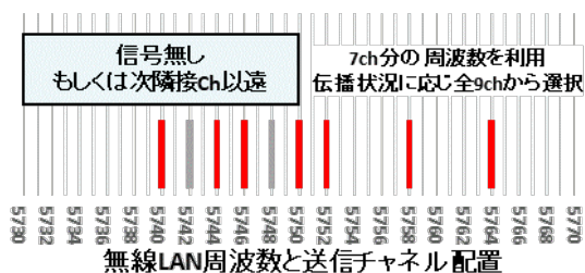
図 2. 2. 12 5. 7GHz 帯におけるチャンネル配置例
