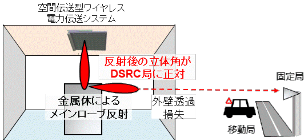
図参 6.2.1 狭域通信システムとの共用検討モデル
