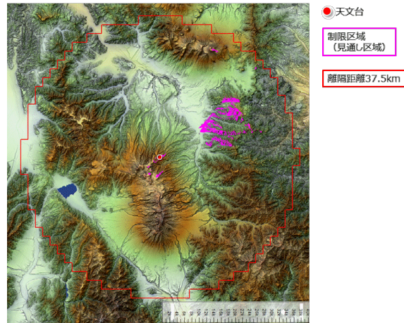
図 3. 3. 2 臼田観測所における空間伝送型ワイヤレス電力伝送システムの制限区域
