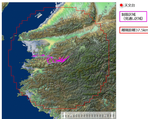
図 3. 3. 3 みさと天文台観測所における空間伝送型ワイヤレス電力伝送システムの制限区域
