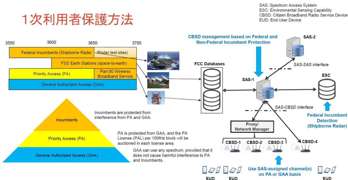
図1 SAS (Spectrum Access System) のシステム構成
