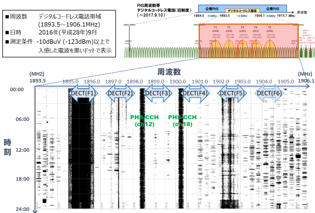
図1. 5-2 デジタルコードレス電話周波数帯域における電波の発射状況(平日24時間、さいたま市浦和区)
