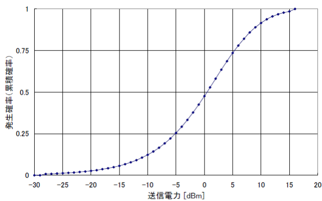
参図 2-23 小電力レピータ 基地局対向器 送信電力分布
