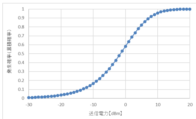
参図 2-7 sXGP 子機送信電力分布
