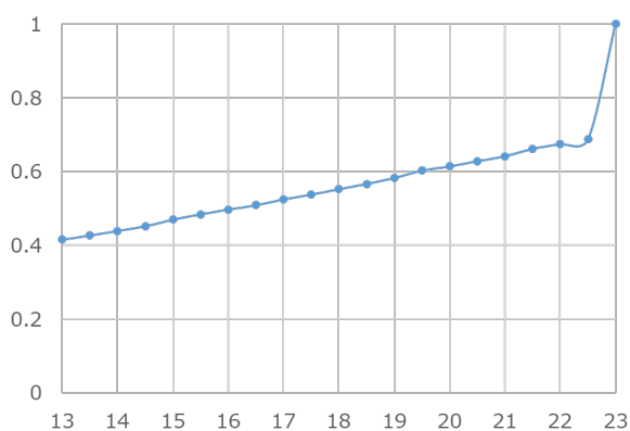
参図 2-6 sXGP 親機送信電力分布
