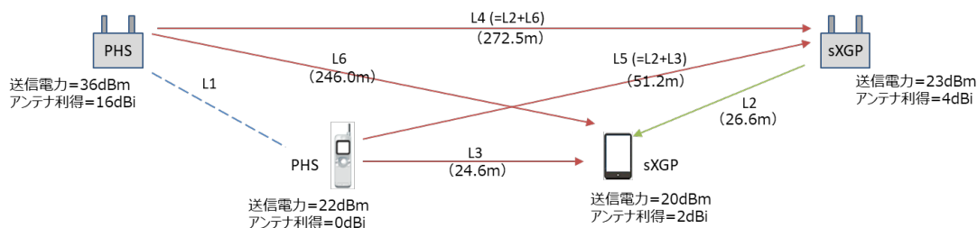
図 2. 2 公衆 PHS 通話チャンネルに対するキャリアセンス値算出モデル
