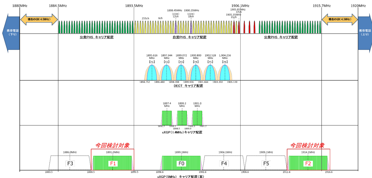
図 2. 1 1.9GHz 帯全体の周波数配置
