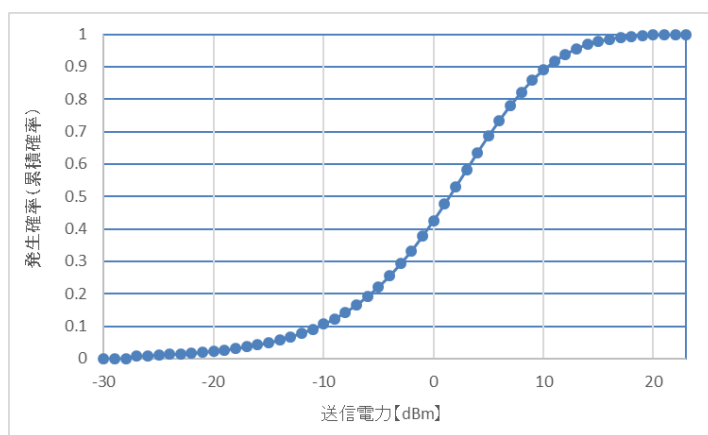
参図 2-22 移動局 送信電力分布
