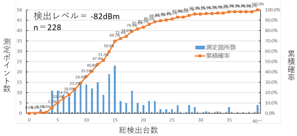
図1. 5-3 住宅地における DECT 方式の親機 ID 検出台数 (福岡市)
