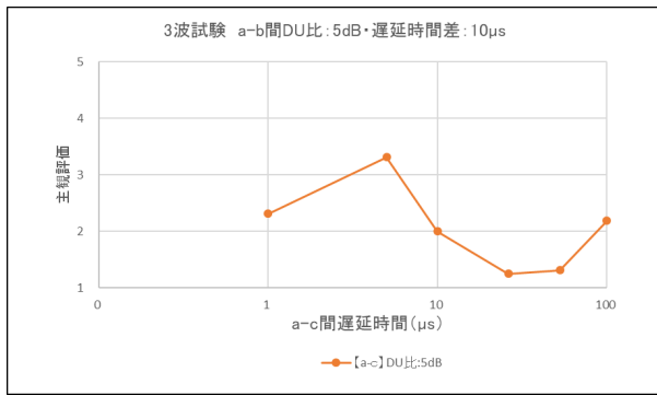
図 3. 2-13 (e) a-b 間 DU 比 5dB ・ 遅延時間差 10 \mu s における 3 波目の影響
