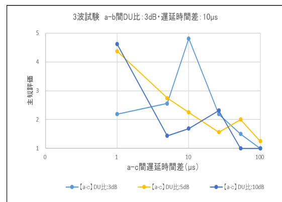
図3.2-13(c) a-b間DU比3dB・遅延時間差10μsにおける3波目の影響
