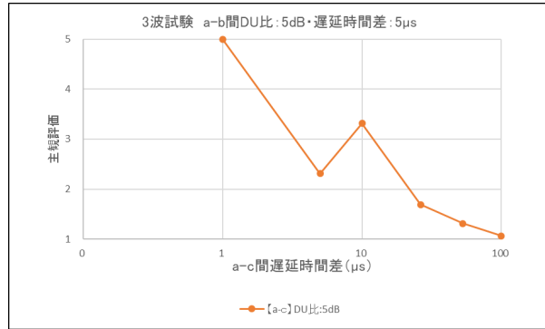
図 3. 2-13 (d) a-b 間 DU 比 5dB ・ 遅延時間差 5 \mu s における 3 波目の影響
