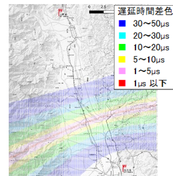
遅延時間差分布の例
