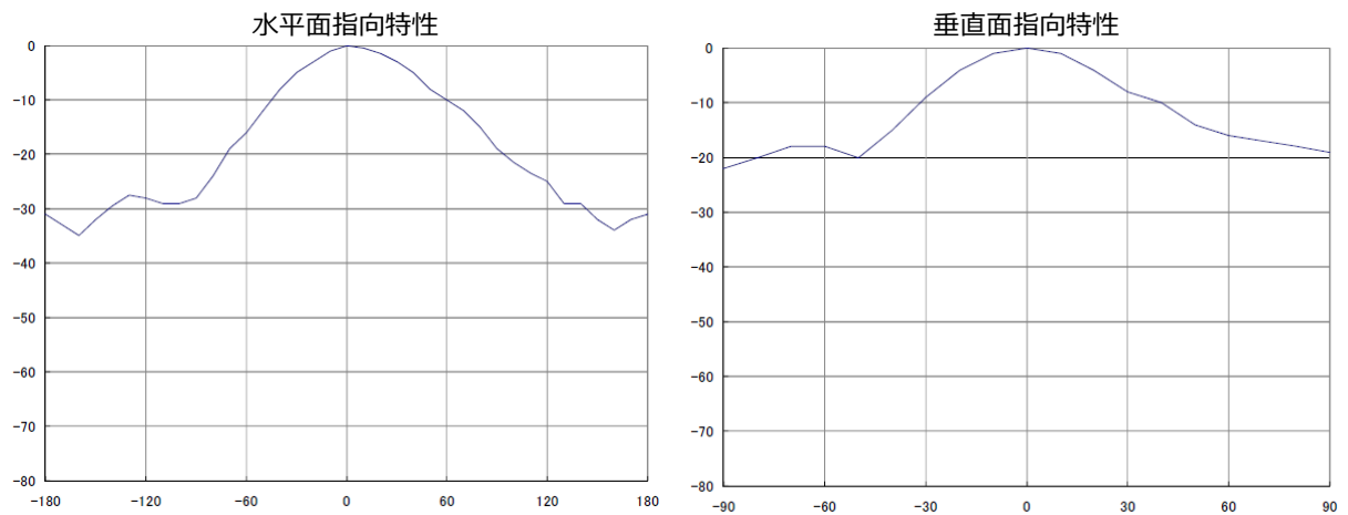
参図2-21 陸上移動中継局 基地局対向器 屋内型 アンテナ指向特性
