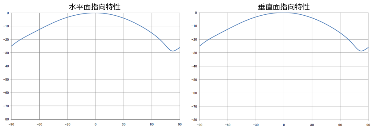
参図2-19 小電力レピータ 基地局対向器 アンテナ指向特性
