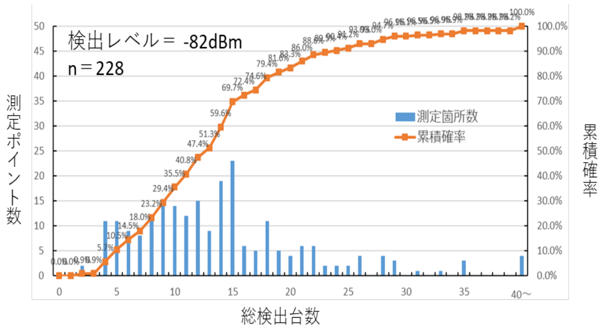
図 1. 5-5 住宅地における DECT 方式の親機 ID 検出点数 (福岡市)
