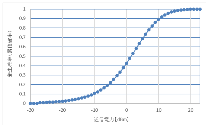
参図2-22 移動局 送信電力分布
