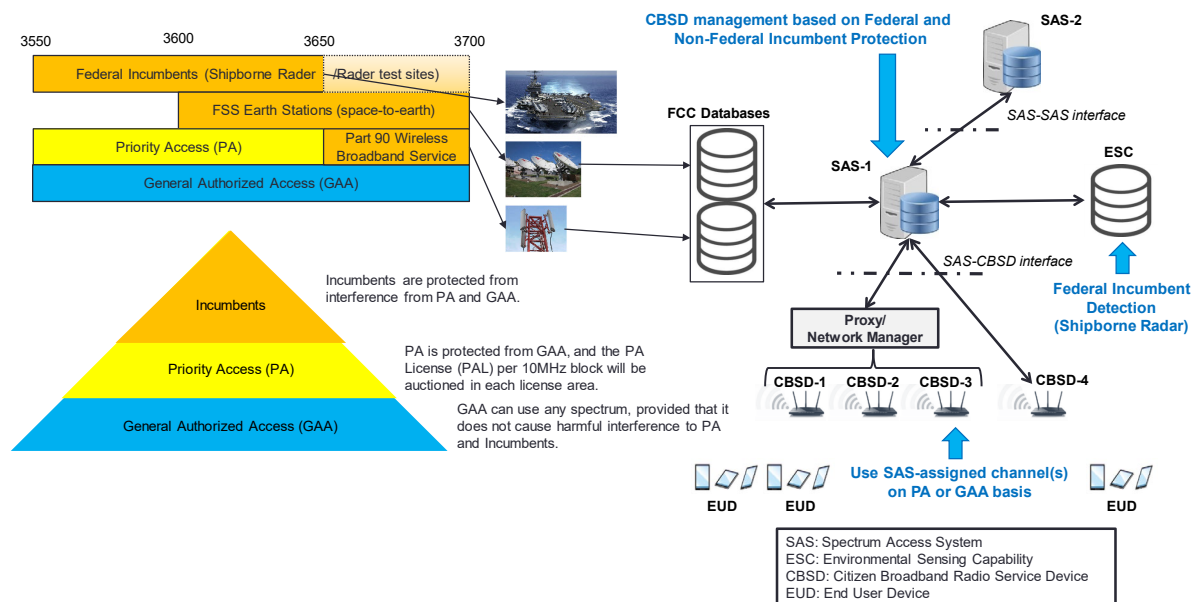
図 1. 4-2 米国の CBRS で用いられている動的な周波数共用技術
