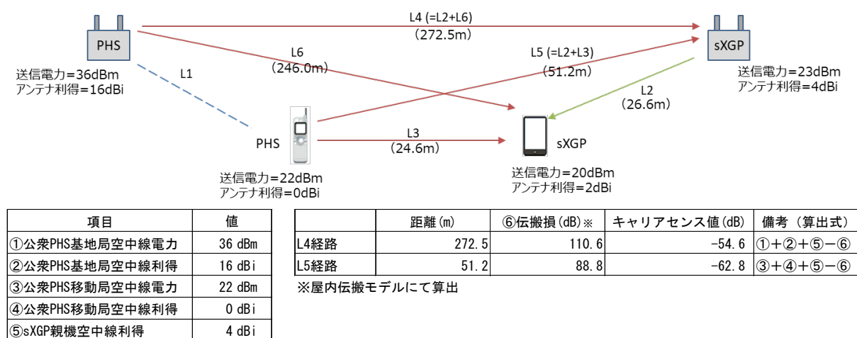
図 2. 3 - 1 公衆 PHS の通話チャネルに対するキャリアセンス値算出モデル
