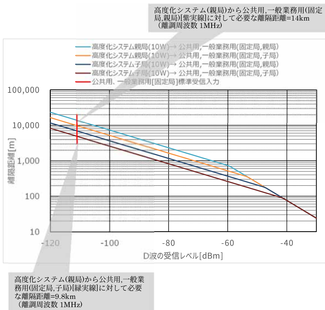
図 2-16 U 波出力 10W (対 公共用、一般業務用[固定局]) + 離調周波数 1MHz
