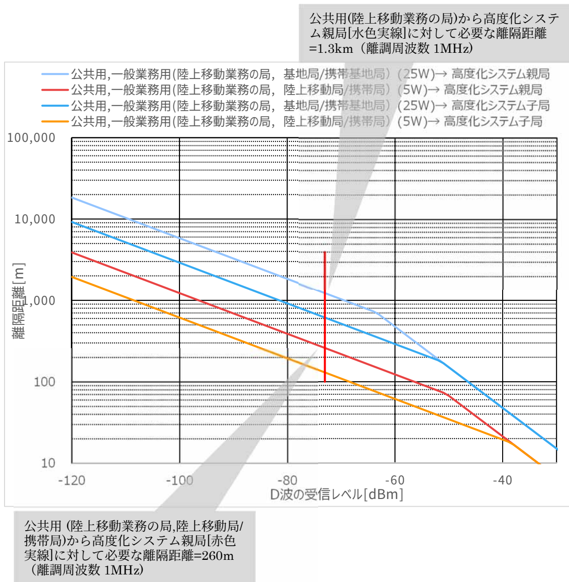
図 2-23 U 波 (対 公共用、一般業務用（陸上移動業務の局）) + 離調周波数 1MHz
