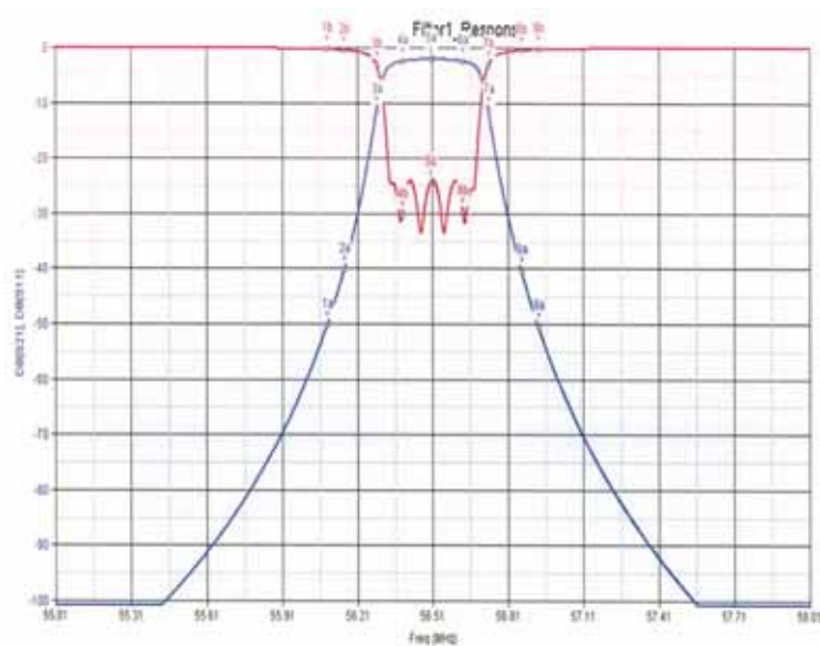
図 6-2 チャンネルフィルタ特性
