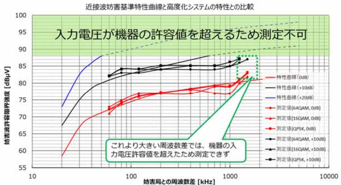
図 8-2 近接波妨害特性の測定結果
