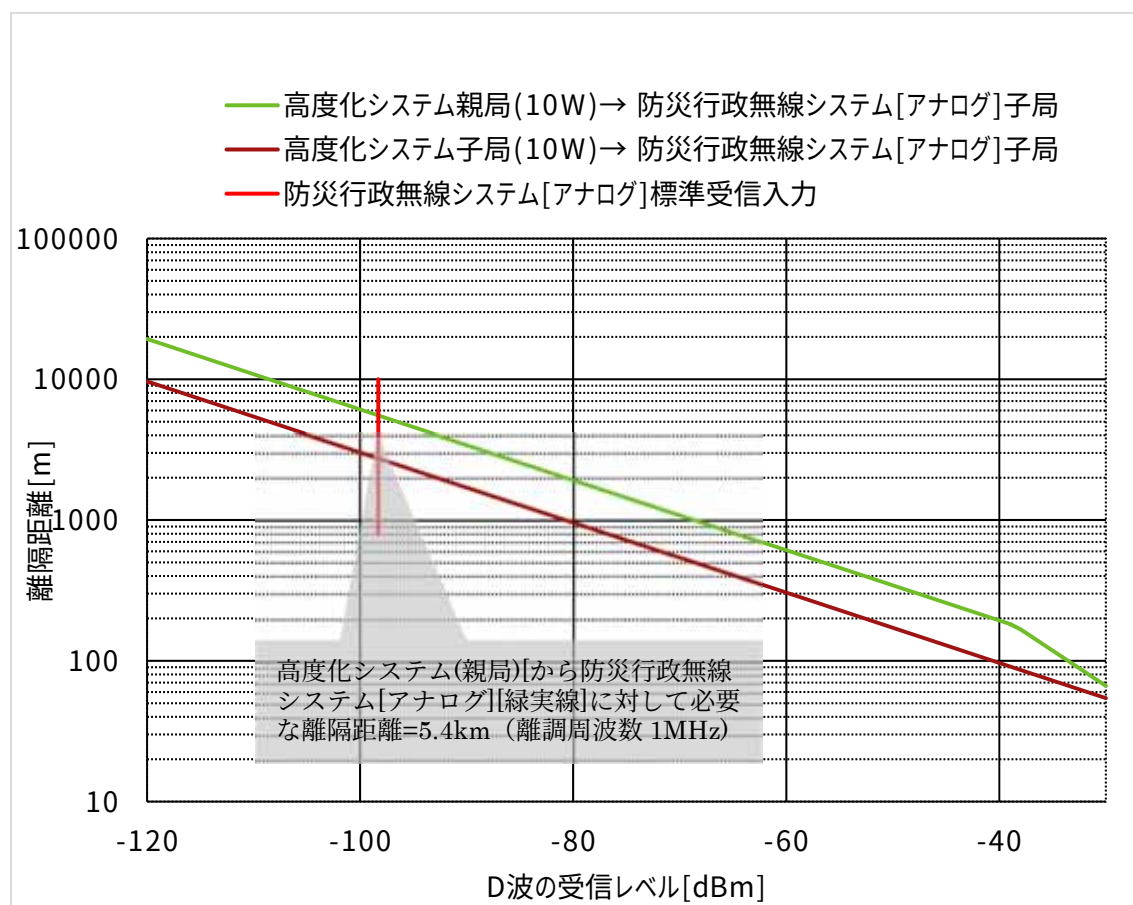
図 2-15 U 波出力 10W (対 防災行政無線システム[アナログ]) + 離調周波数1MHz
