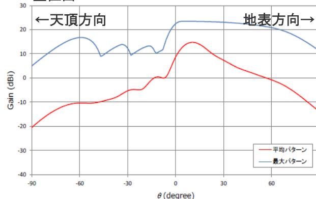
マクロセル局の空中線指向特性(チルト6度)
