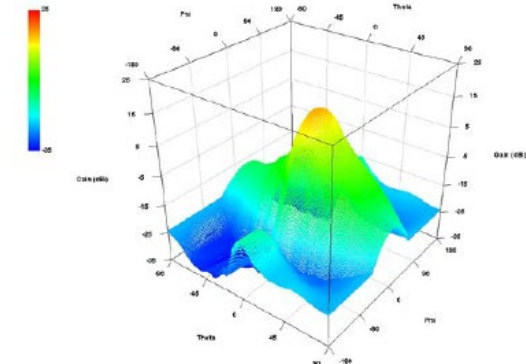
(b) 平均パターン
