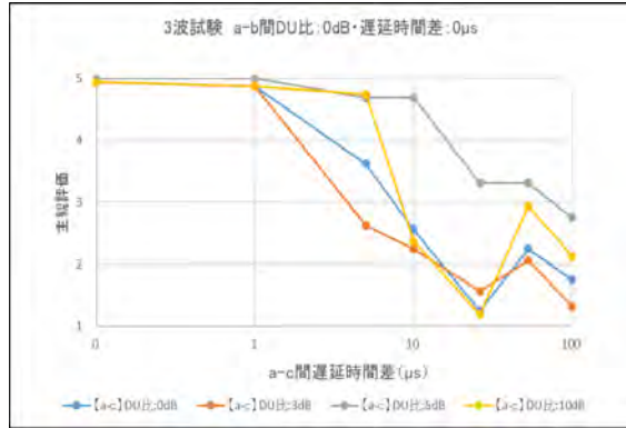
図 3.2-13(a) a-b 間 DU 比 0dB・遅延時間差 0 \mu\text{s} における 3 波目の影響
