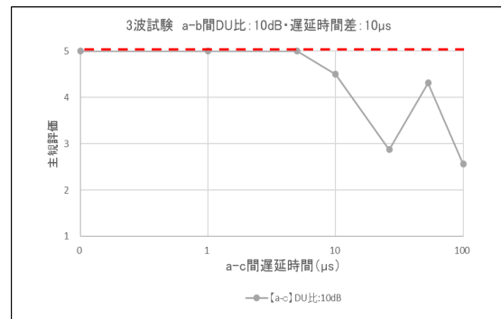
図 3. 2-14 (g) a-b 間 DU 比 10dB・遅延時間差 10 \mu\text{s} における 3 波目の影響
