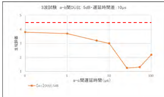
図 3. 2-14 (e) a-b 間 DU 比 5dB・遅延時間差 10 \mu\text{s} における 3 波目の影響
