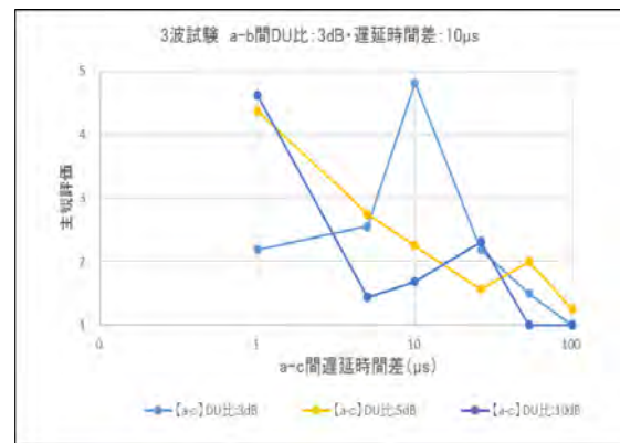
図 3.2-13(c) a-b 間 DU 比 3dB・遅延時間差 10 \mu\text{s} における 3 波目の影響
