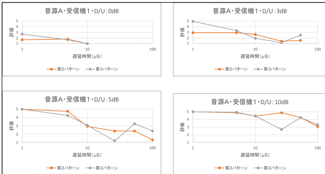
図 3.2-15 第3パターン、第2パターンの比較
