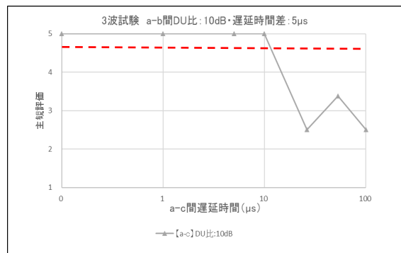
図 3. 2-14 (f) a-b 間 DU 比 10dB・遅延時間差 5 \mu\text{s} における 3 波目の影響
