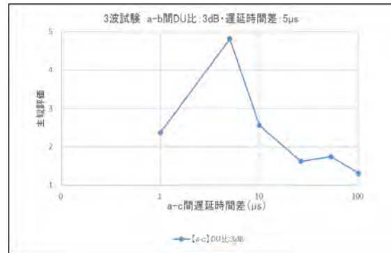
図 3.2-13(b) a-b 間 DU 比 3dB・遅延時間差 5 \mu\text{s} における 3 波目の影響
