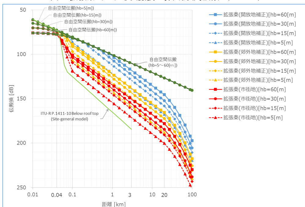
図 1 拡張秦式による伝搬損失の算出例 (周波数=2,585MHz)
