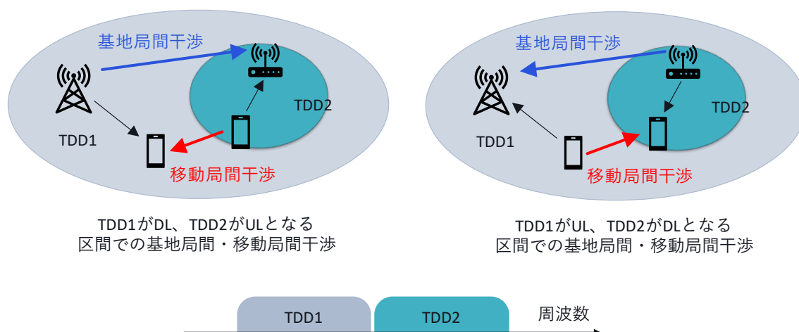
図3. 2. 2 隣接等周波数を用いる TDD 1（全国5 G）と TDD 2（ローカル5 G）の基地局間・端末間干渉
