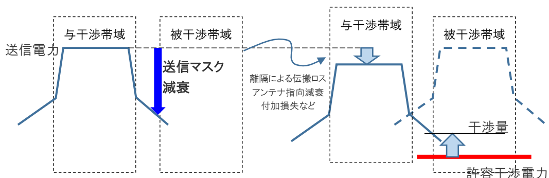
図4. 2. 1. 2-4 最悪値条件による干渉計算のイメージ（隣接周波数を使用する5G相互間）
