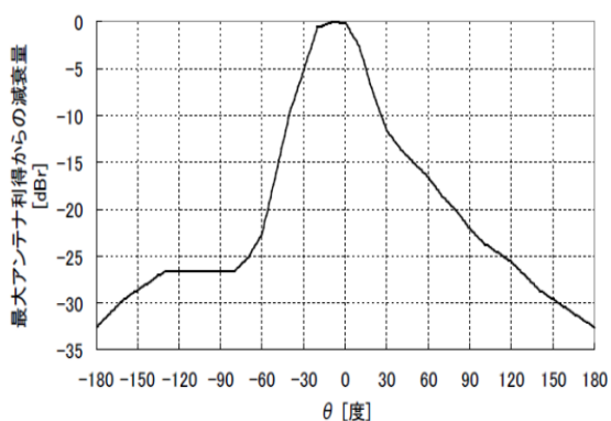
移動衛星(N-STAR移動局) 垂直面 (P62 参図3.1)
