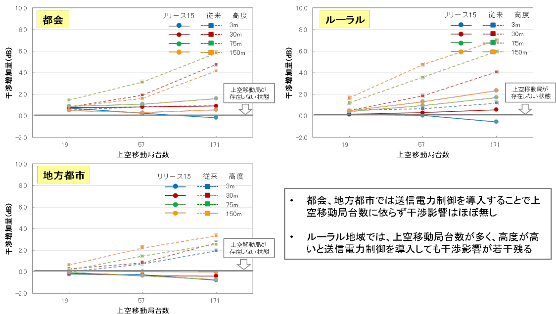
図2. 1. 3-3 2.5GHz帯におけるシミュレーション結果
