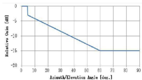
ITU-R SA.1165-2 (P192 図 参考1-2-1)
