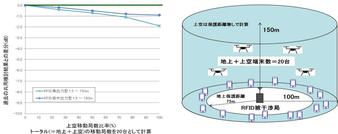
図2. 3. 4－6 RFID との共用検討結果（確率計算）
