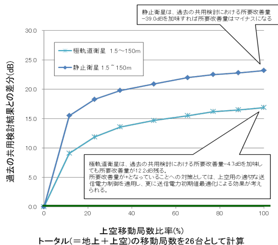
図 2. 3. 4-7 気象衛星 (↓) との共用検討結果 (確率計算)
