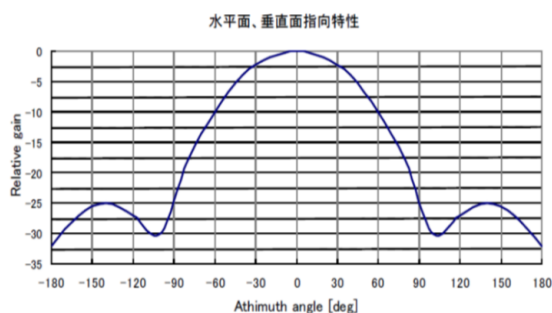
RFID高出力型パッシブタグシステム(垂直、水平面) (P456図、参1-8-1)
