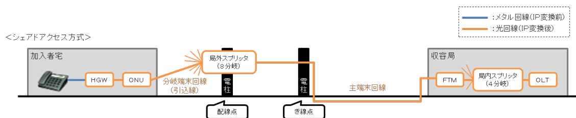
図5-4 シェアアクセス方式
