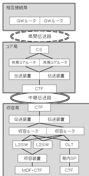
図5-14 各設備の冗長構成(伝送装置にPTNを用いる場合)
