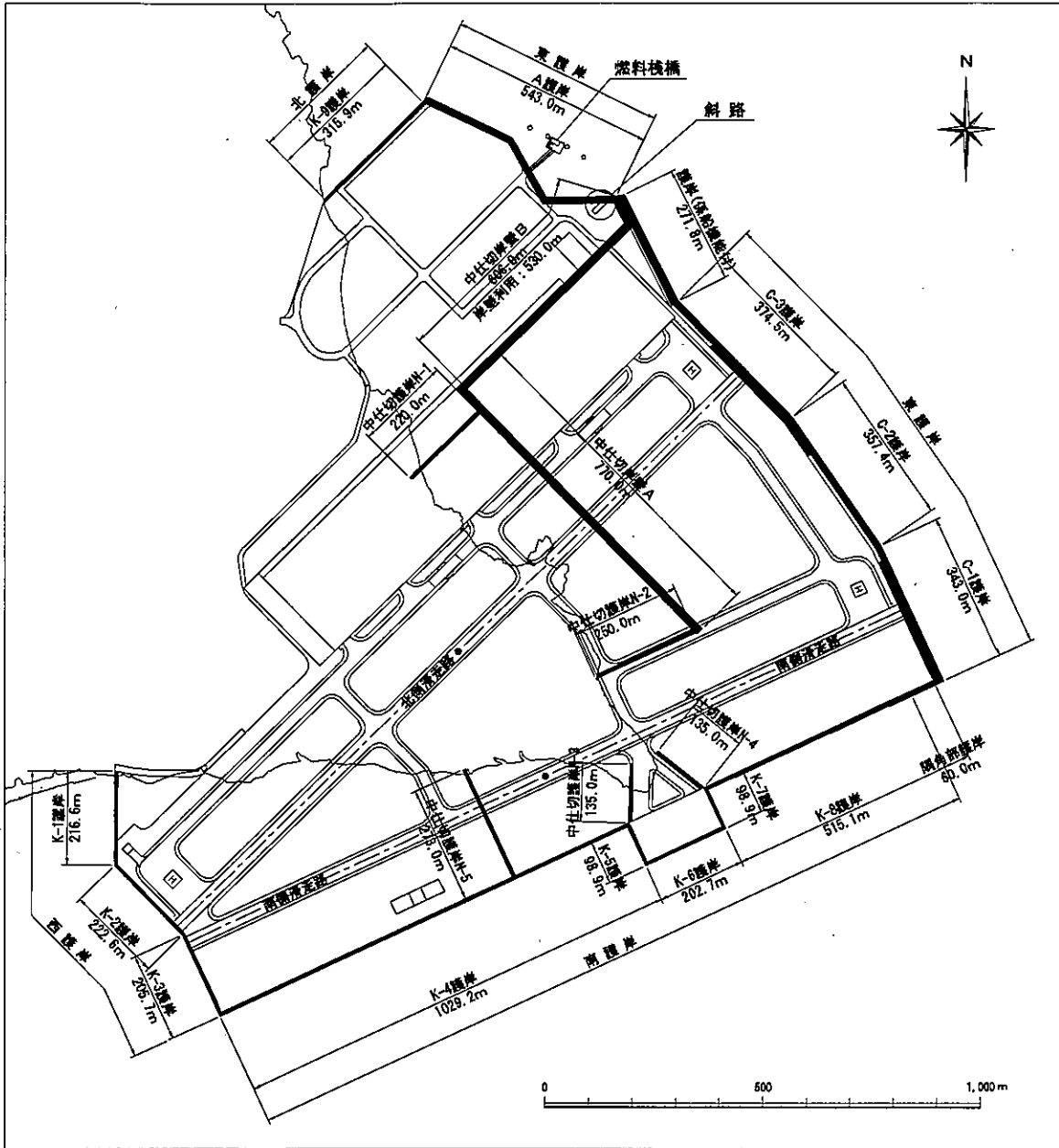
図 2.1.1 工作物の配置及び施行延長【変更後】
