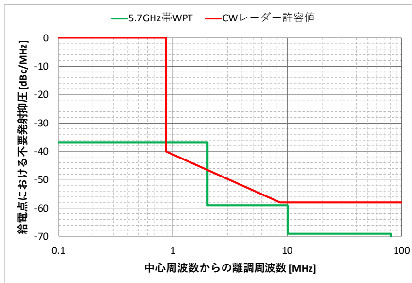
図参 13.4.1 5.7GHz 帯の不要発射の強度の許容値比較
