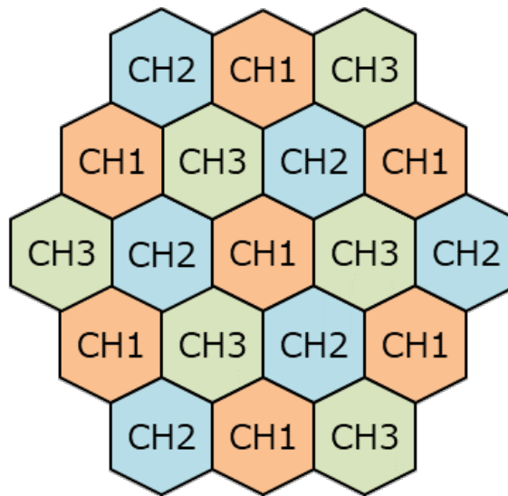
図 2.2.9 920MHz 帯のチャンネル使用例（当初検討）
