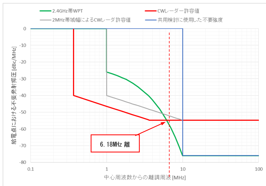
図参 13.3.1 2.4GHz 帯の不要発射の強度の許容値比較
