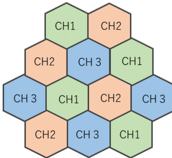
図 2. 2. 11 2. 4GHz 帯におけるチャネル配置例
