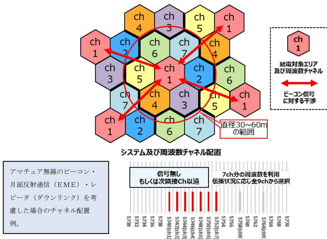
図 2. 2. 12 5. 7GHz 帯におけるチャンネル配置例
