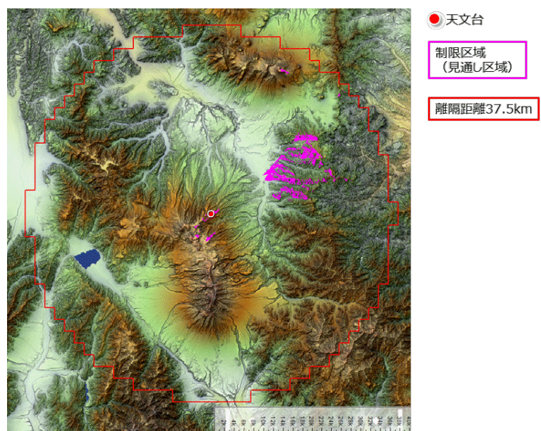
図参 4. 4. 3 臼田観測所における空間伝送型ワイヤレス電力伝送システムの制限区域
