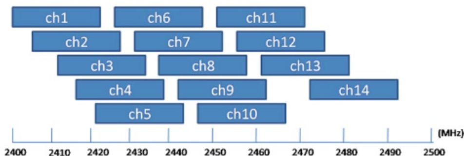
図 3.1.3 2.4GHz 帯無線 LAN システム (IEEE802.11b : 20MHz システム) のチャネル配置
