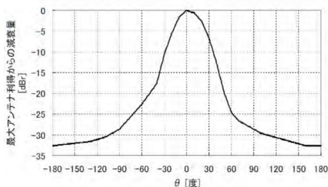
図参 1. 2. 2 水平面内指向特性
