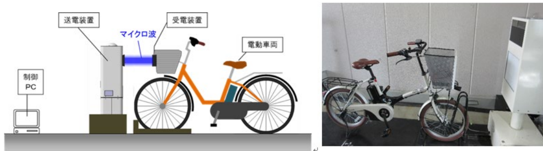
図 1.1.4 電動車両向け空間伝送型ワイヤレス電力伝送システムの社会実証実験（イ）
