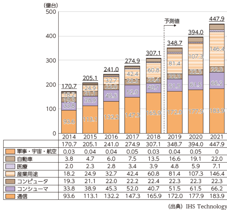
図 1. 4. 1 世界の IoT デバイス数の推移及び予測※3
