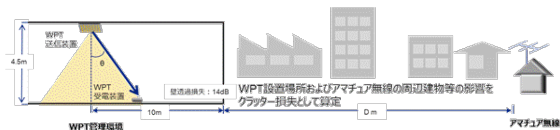
図参 5.9.1 アマチュア無線との共用検討モデル
