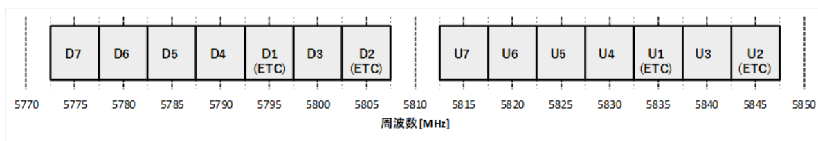
図 3.1.6 DSRC におけるチャネル配置
