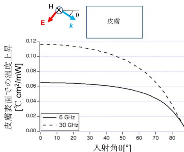
図4. 表面温度上昇の入射角依存性（ 1\text{mW}/\text{cm}^2 垂直偏波入射時）[8]
