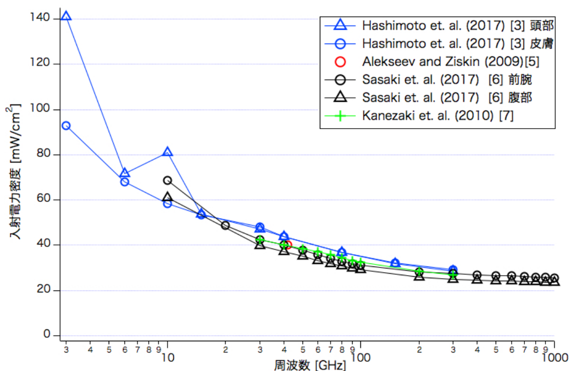
図5. 5℃の温度上昇を得るために必要な入射電力密度（[3] [5] [6] [7]に基づく）
