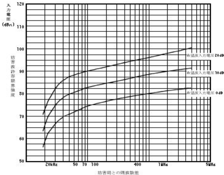
電波法関係審査基準別図第37号の2を抜粋
