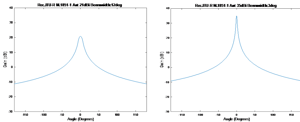
(アンテナ特性-2)
