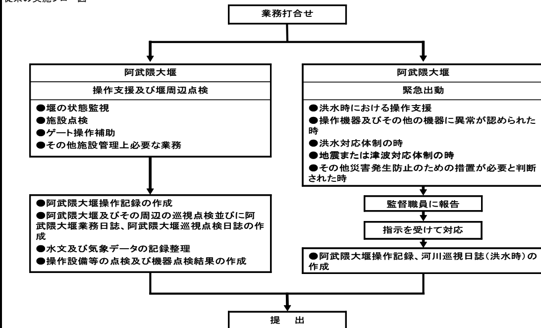
従来の実施フロー図
