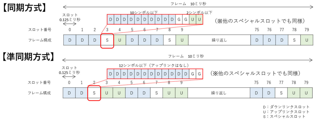
図 2 28.2~29.1GHzの周波数帯における送信装置のフレーム構成
