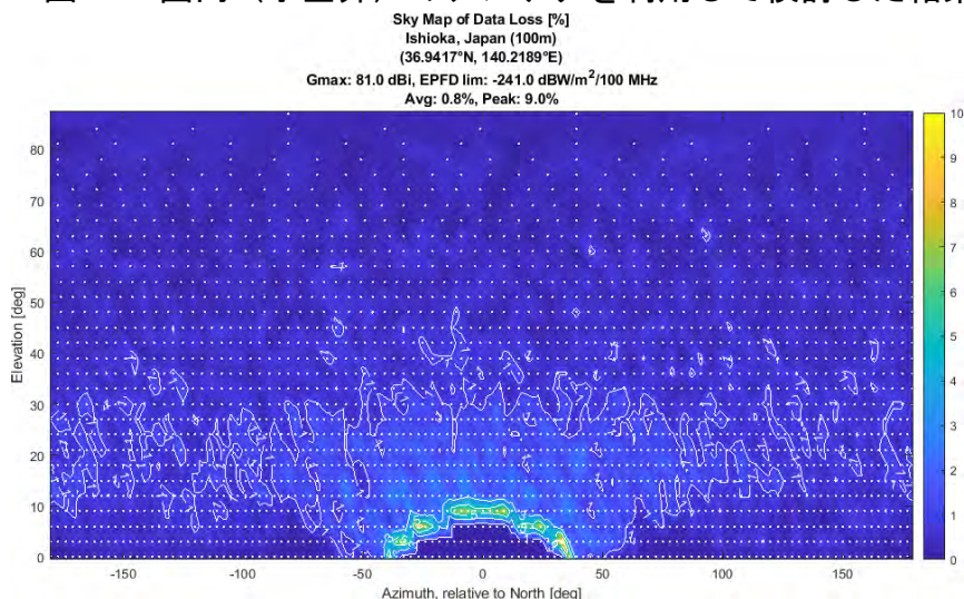
図 2-5 国内（石岡）のアンテナを利用して検討した結果
