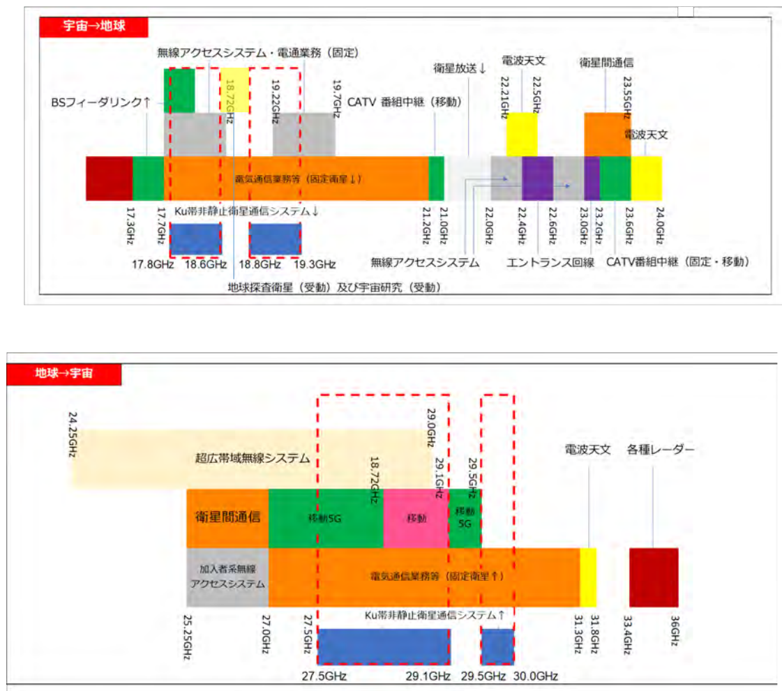
図 2-2 我が国における Ka 帯の周波数使用状況
