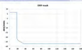
図 参1-1 地球局パラメータ
