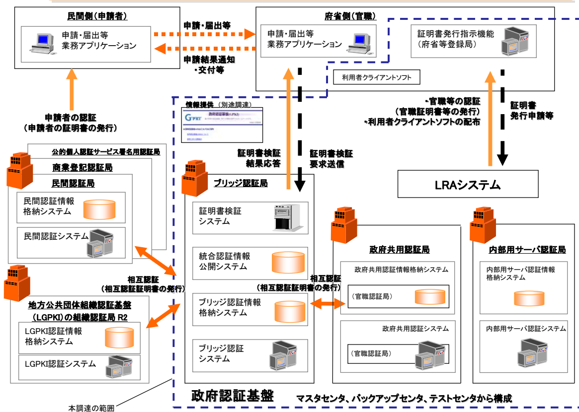
図 2-2 政府認証基盤システムの概要
