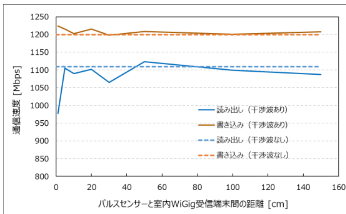
図3-13 実証試験結果(屋内 WiGig システムの通信速度)
