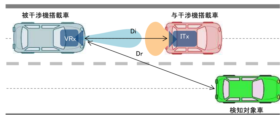
図3-28 干渉検討モデル(自動車レーダー)
