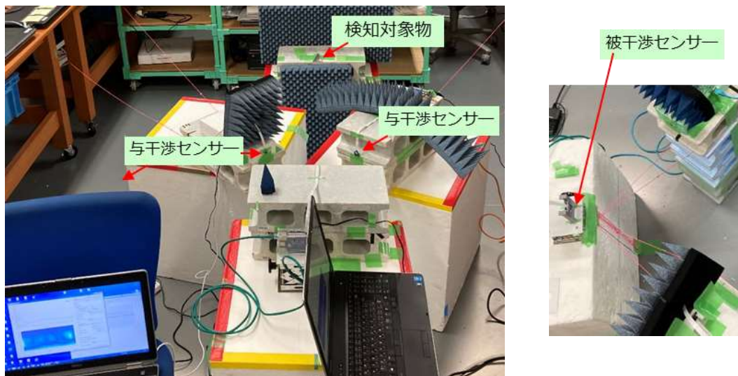
参考図4-4 実験の様子(パルスセンサー同士の干渉)
