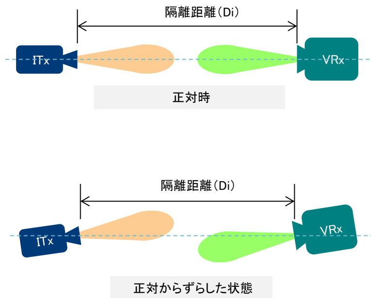
図3-35 干渉検討モデル(固定局)
