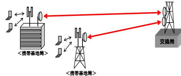
固定通信システム(携帯基地局エントランス)
