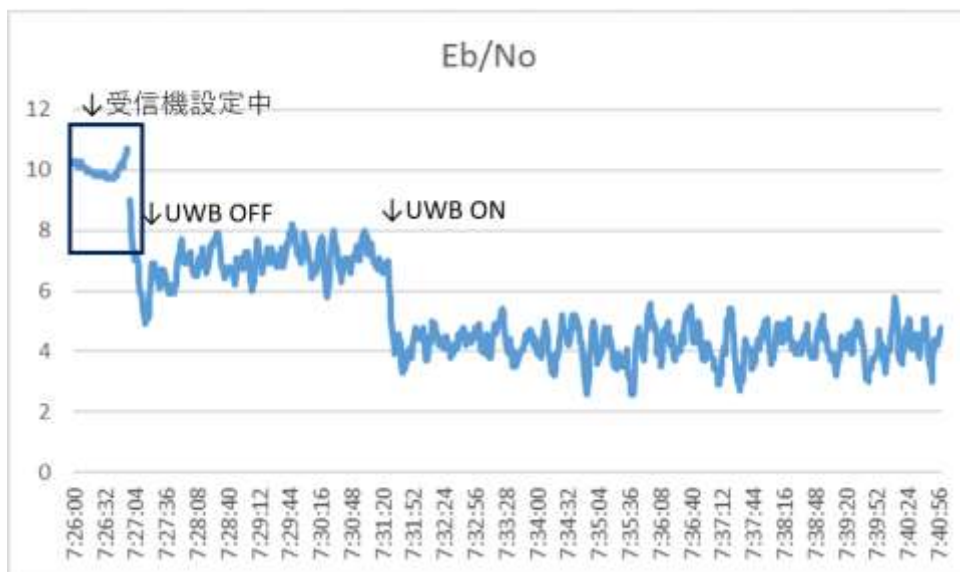
図6-3 Eb/Noの影響
