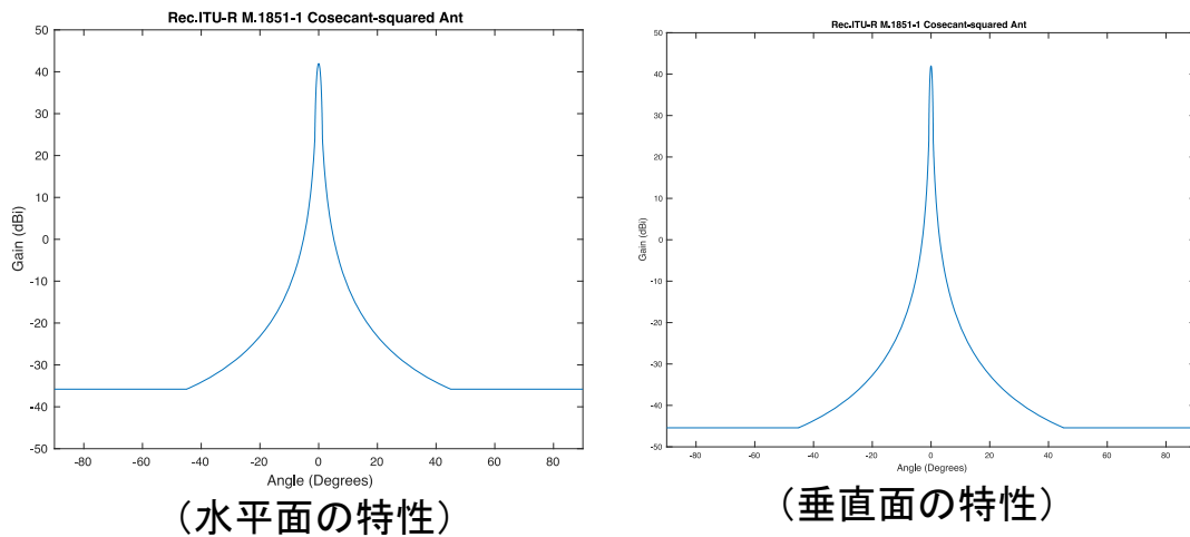
図 3-9 航空機精測進入レーダー（PAR）のアンテナ特性
