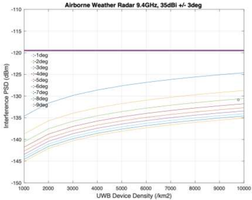
図5-19 高度1050m条件での計算結果（アンテナ特性2）
