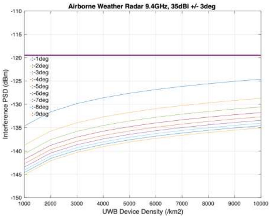
図5-18 高度520m条件での計算結果（アンテナ特性2）
