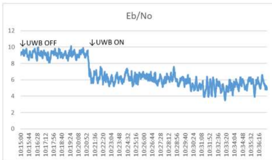
図6-7 Eb/Noの影響
