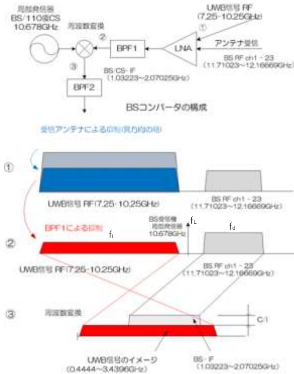
図 3-20 UWB イメージ信号と BS/CS 放送の IF 周波数の関係
