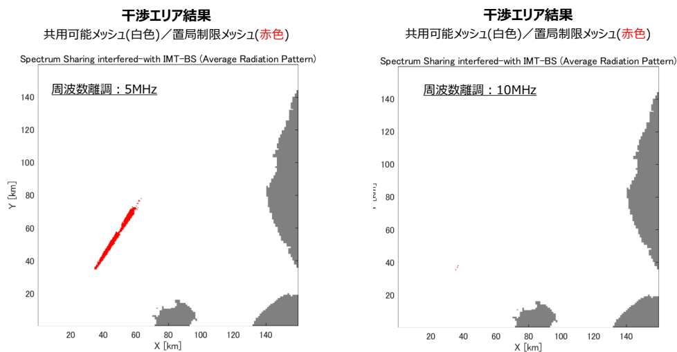
図 3. 4-15 周波数離調
