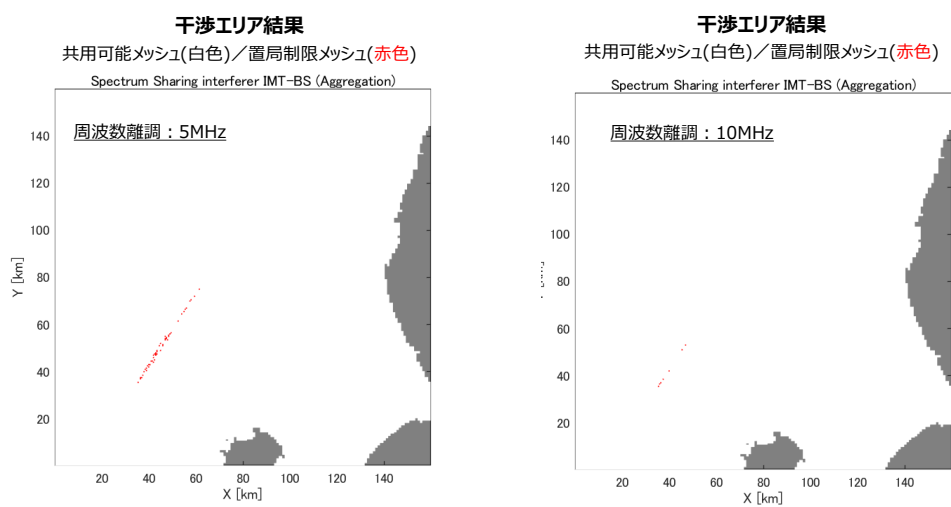
図 3. 4-24 周波数離調
