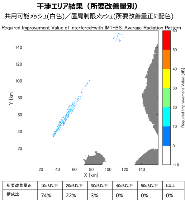
図 3. 4－27 隣接チャネル共用計算結果（周波数離調なし）：所要改善量別
