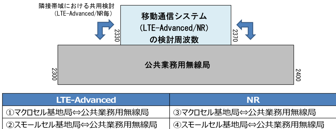
図 3. 4-2 移動通信システムと公共業務用無線局の干渉検討パターン
