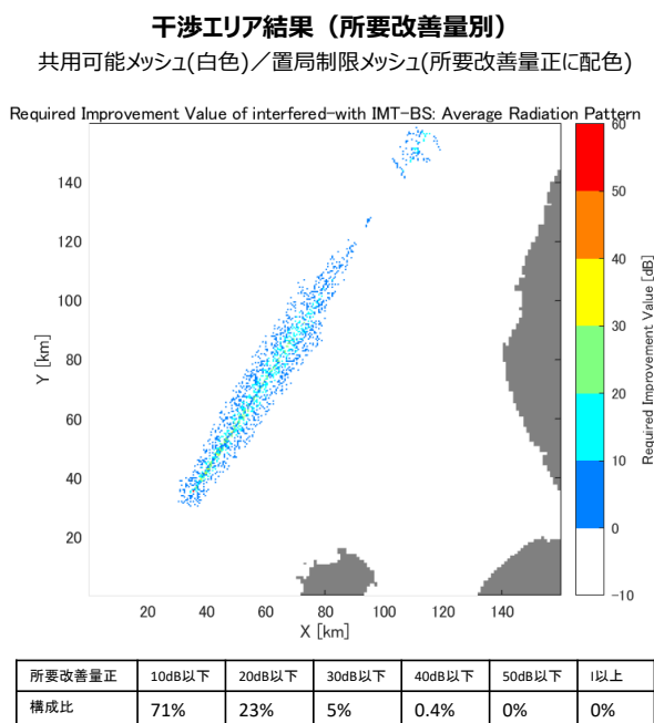
図 3. 4-20 隣接チャネル共用計算結果（周波数離調なし）：所要改善量別
