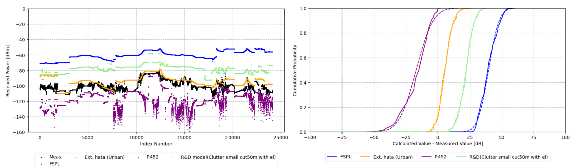
図 参考 1- 6 測定結果と電波伝搬モデル対比（都市部・全体）
