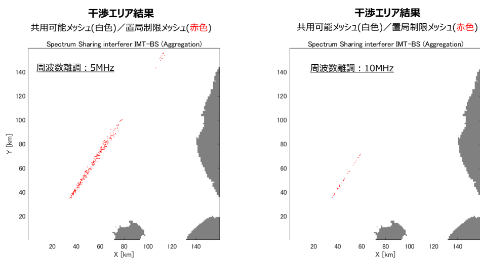
図 3. 4-17 周波数離調
