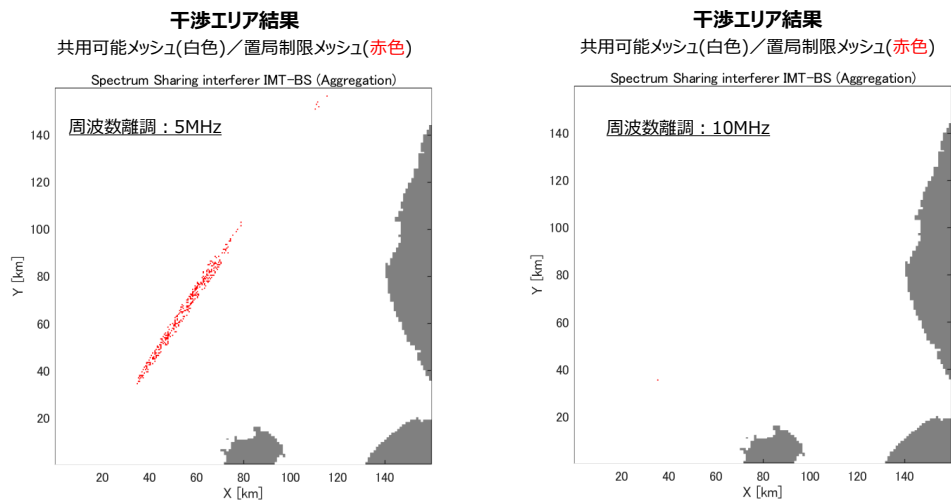
図 3. 4-4 周波数離調
