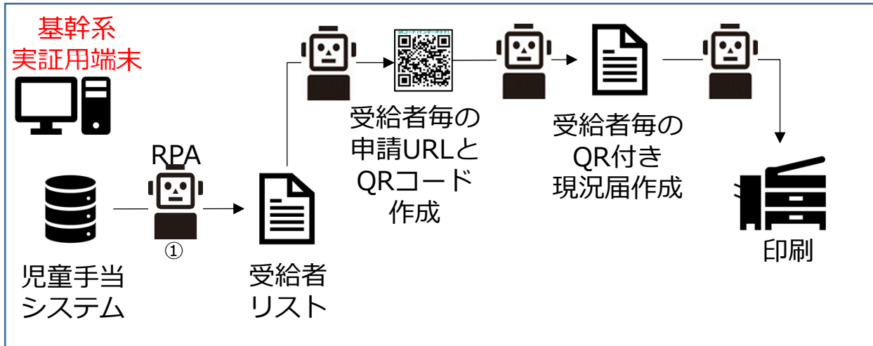
図4.5.4 導入モデル_システム図
