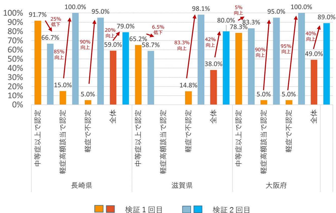
一次審査（AI自動判定）認定結果との一致率（検証1回目と2回目比較）
