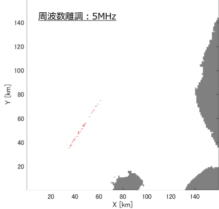
図 3. 4-28 周波数離調
