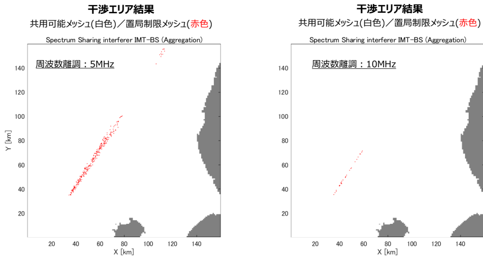
図 3. 4-17 周波数離調
