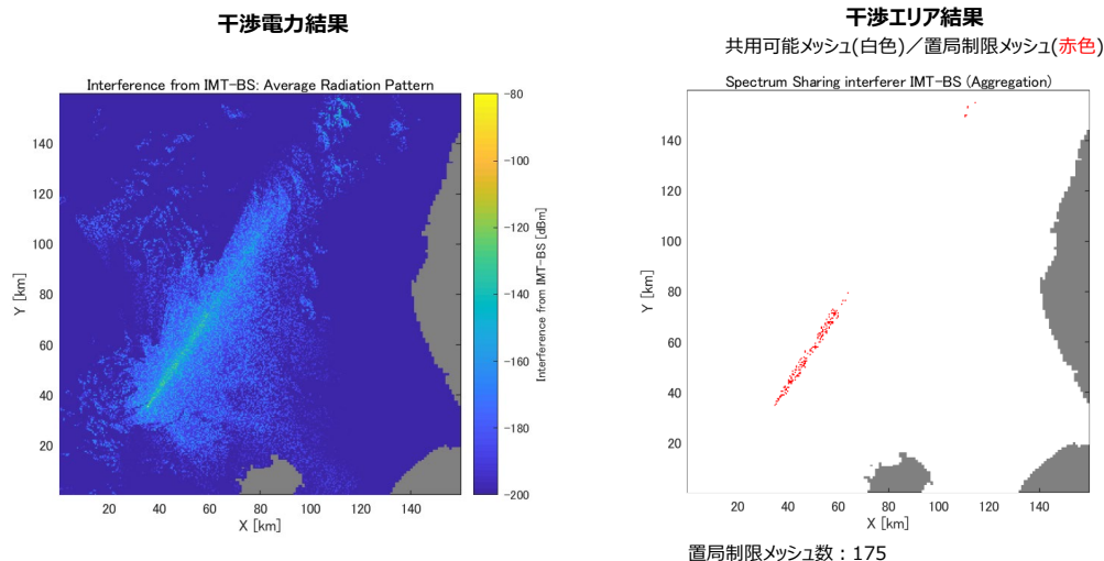
図 3. 4-23 隣接チャネル共用計算結果（周波数離調なし）
