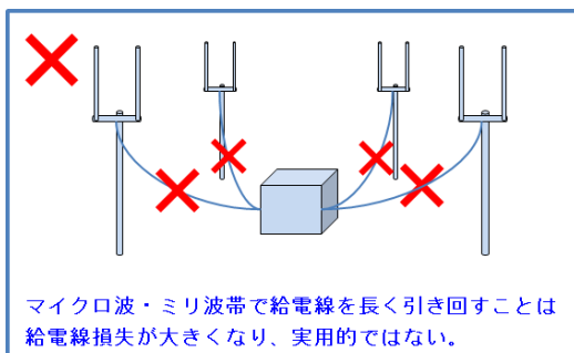
図 2. 3. 2. 3-2 複数の空中線設置
