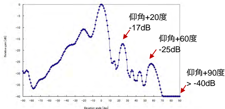
図2. 2. 1-2 基地局の送受信アンテナパターン(垂直面) (携帯電話等周波数有効利用方策委員会報告(平成18年12月21日)の図3. 2-2に基づきシミュレーションを用いて仰角10度以上に拡張) 情報通信審議会・情報通信技術分科会・新世代モバイル通信システム委員会「新世代モバイル通信システム委員会報告書」平成29年(2017年)9月27日
