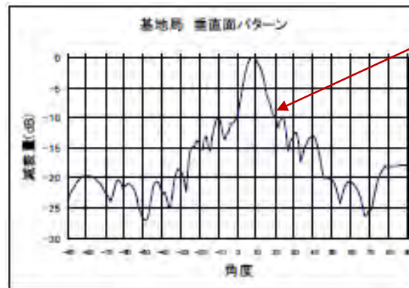
PHS基地局の送受信アンテナパターン（垂直面）
