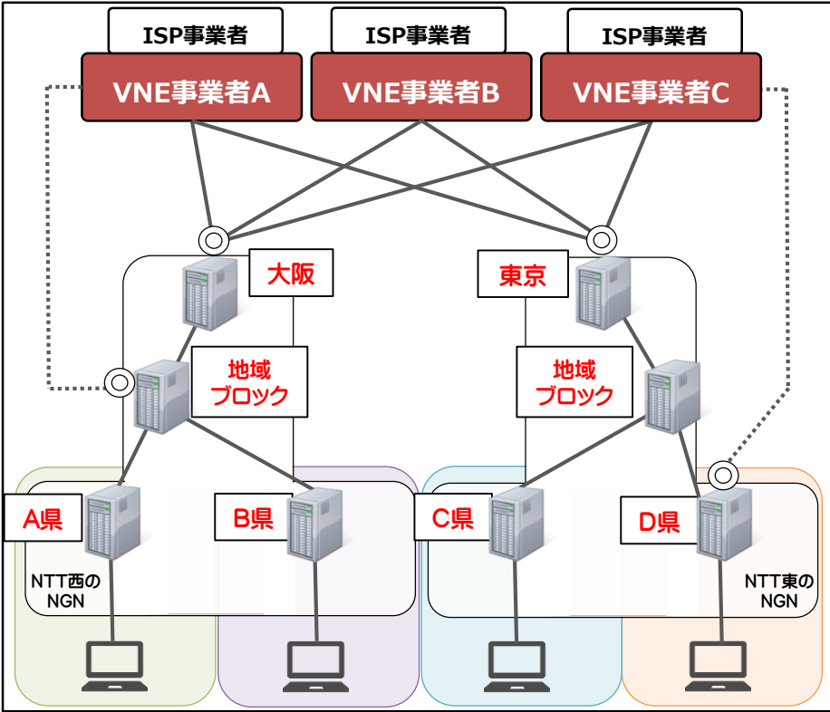
【IPoE接続】
