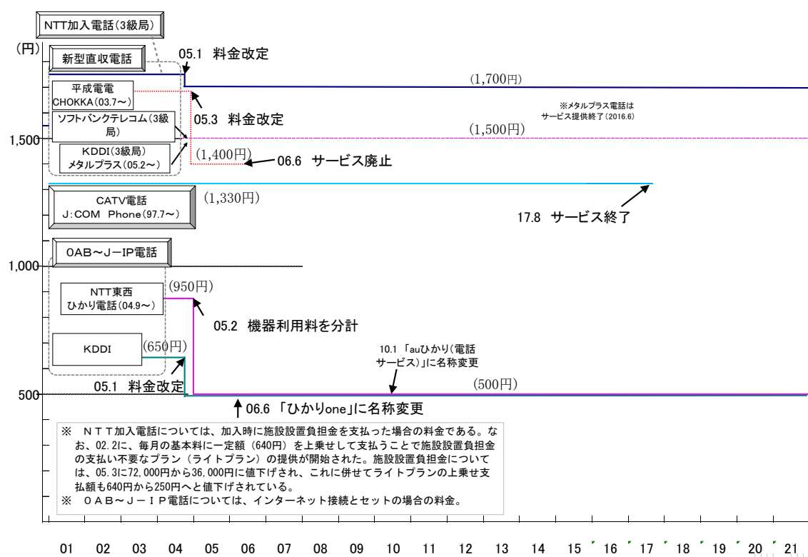
【図表Ⅲ－６】固定電話サービスの基本料金の推移
