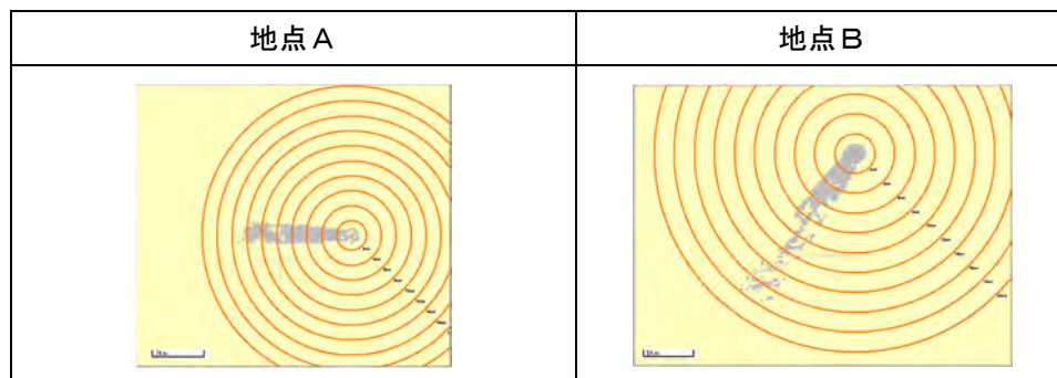
図 参 2-3 移動地球局（水平方向 EIRP -33\text{dBW}/40\text{kHz} ）の干渉エリア
