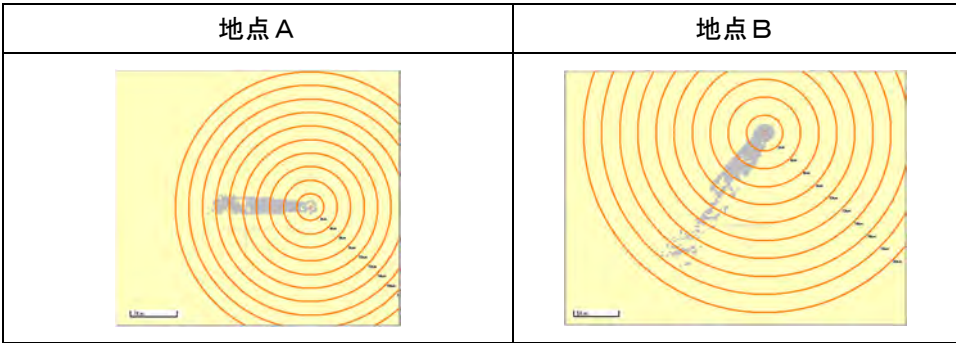
図 2-5 移動地球局 (水平方向 EIRP -33\text{dBW}/40\text{kHz} ) の干渉エリア
