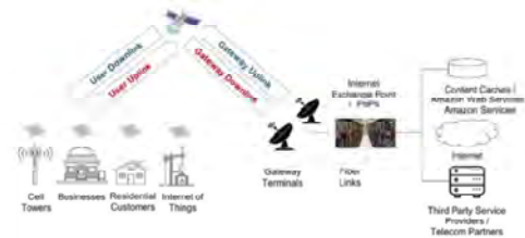
LEO衛星コンステレーションシステム概要
