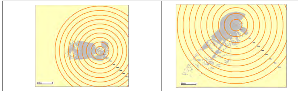
図 2-6 移動地球局（水平方向 EIRP -20dBW/40kHz）の干渉エリア
