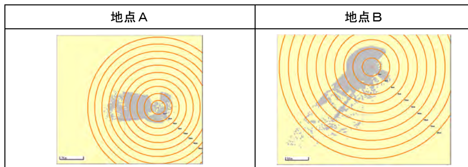
図 参 2-4 移動地球局（水平方向 EIRP -20\text{dBW}/40\text{kHz} ）の干渉エリア
