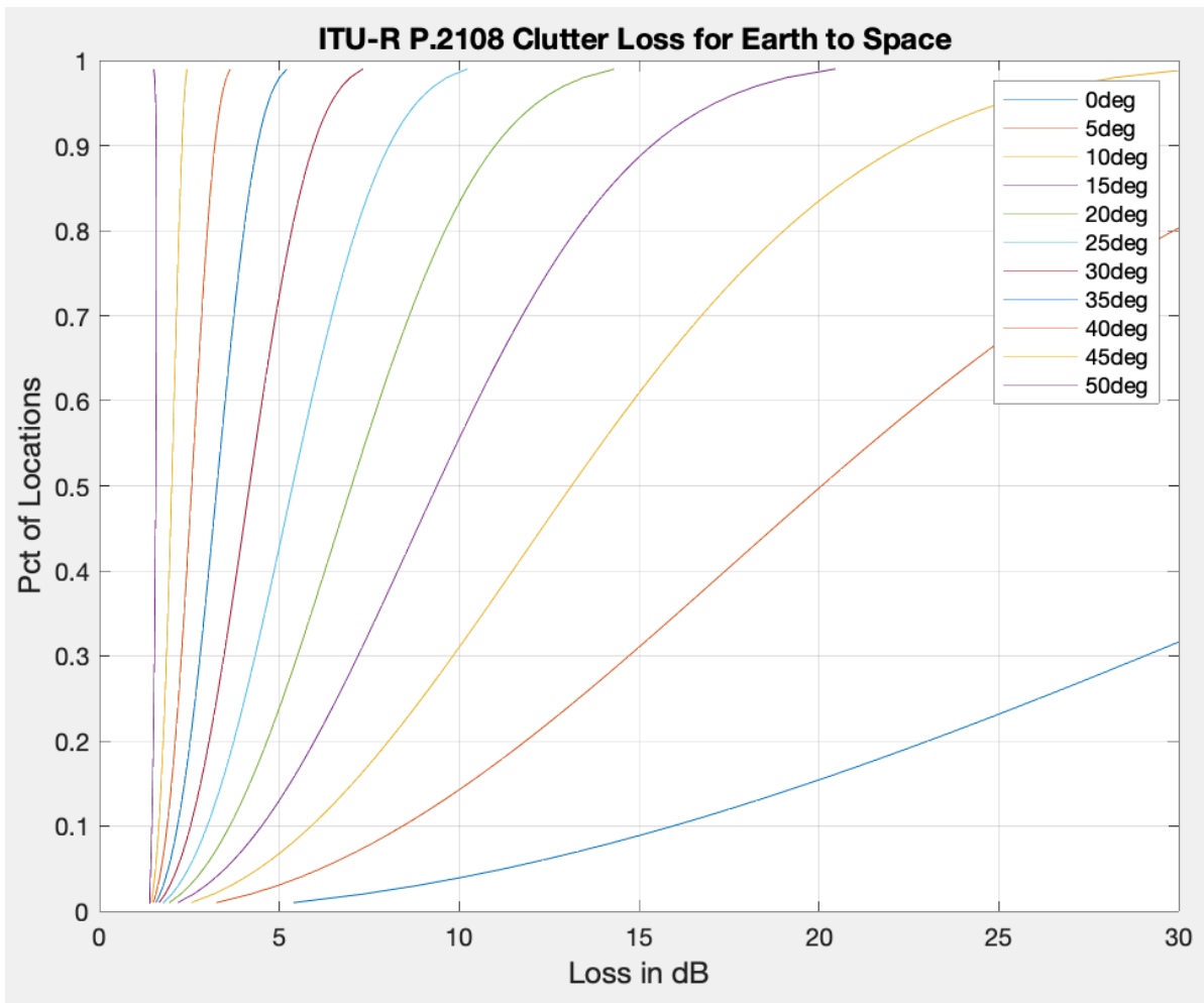
図 5-3-1-2 ITU-R 勧告 P. 2108 によるクラッタ損失
