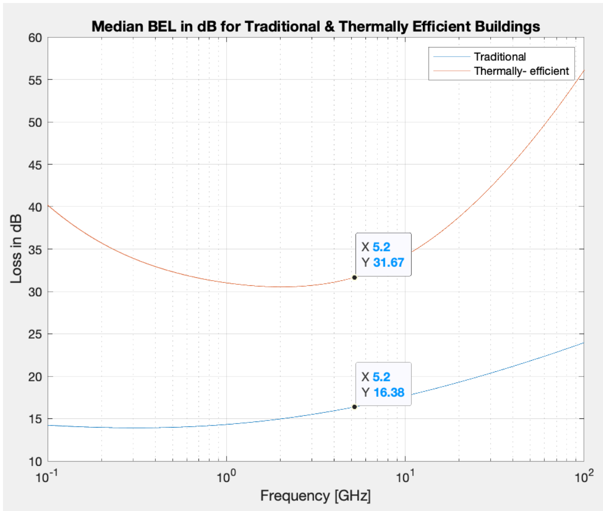
図 5-3-1-1 ITU-R 勧告 P. 2109 による建物遮蔽損失
