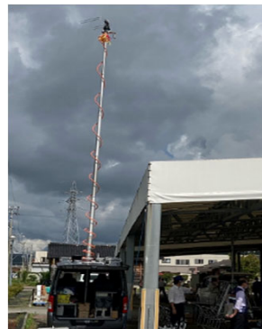
伸縮ポール装備の車両に臨時災害放送局の送信アンテナを設置
