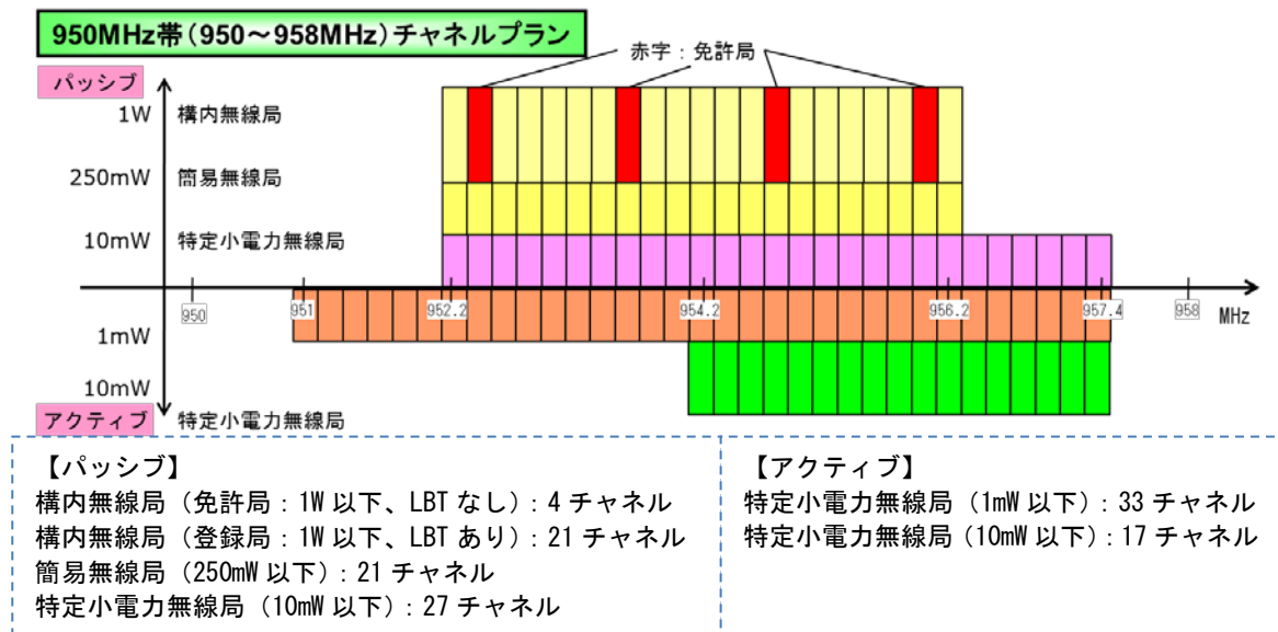
図 4-1 950MHz 帯電子タグシステムのチャネルプラン
