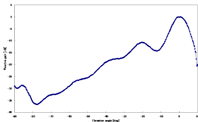
参考図 6-4 CDMA2000 基地局の送受信アンテナパターン(垂直面)
