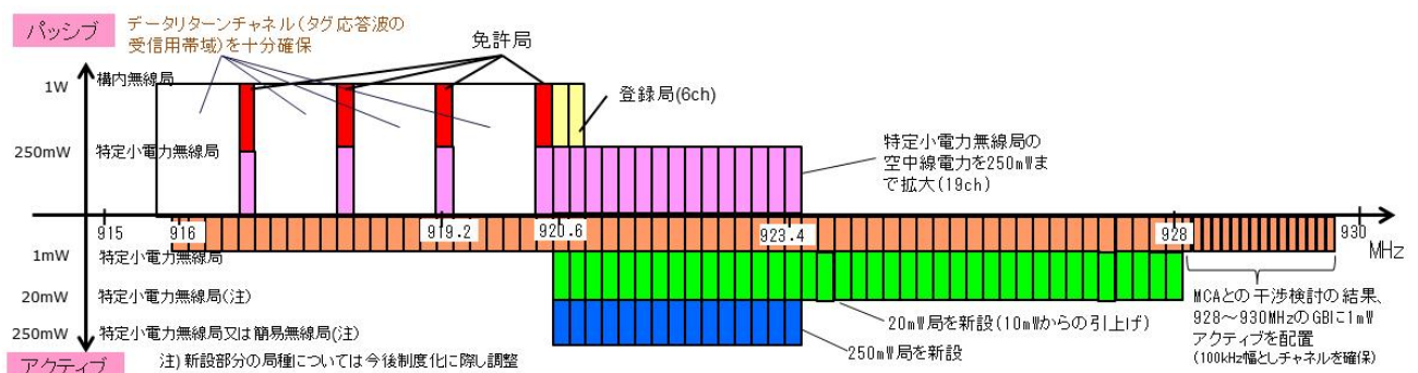
図 4-5 920MHz 帯電子タグシステム等のチャンネルプラン
