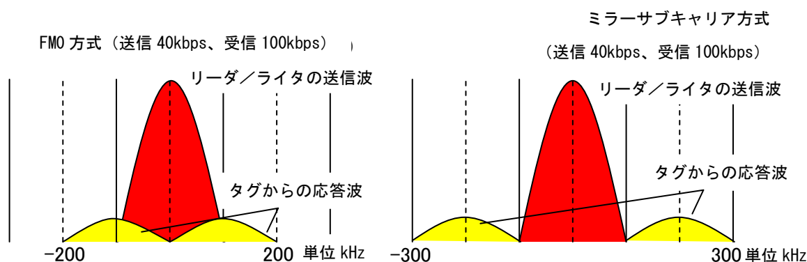
図 4-2 FM0 方式とミラーサブキャリア方式のスペクトル例
