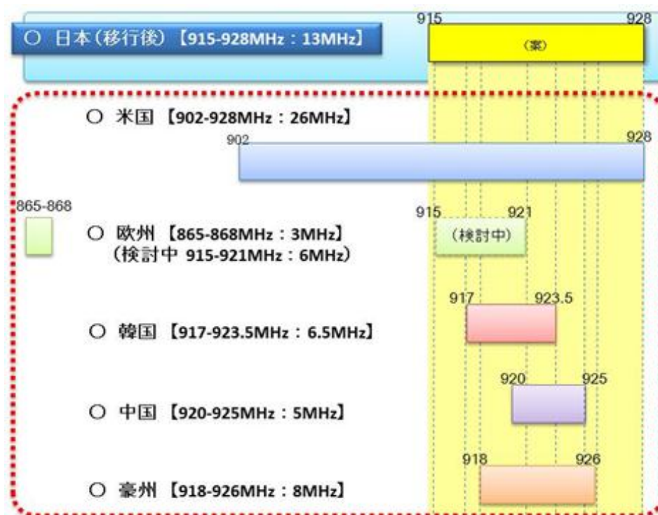
図 4-4 電子タグシステム用途の諸外国における周波数割当状況
