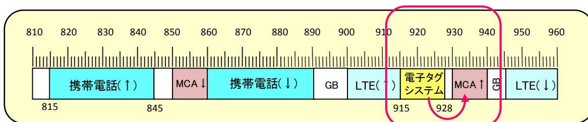
参図 5-1 920MHz 帯の周波数配置 (移行完了後)
