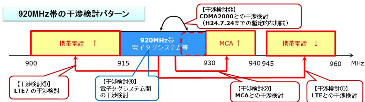
図 5-1 920MHz 帯電子タグシステム等の干渉検討の組み合わせ
