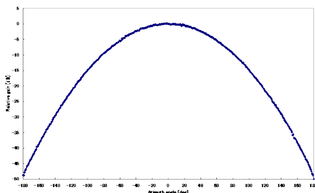
参考図 6-3 CDMA2000 基地局の送受信アンテナパターン(水平面)
