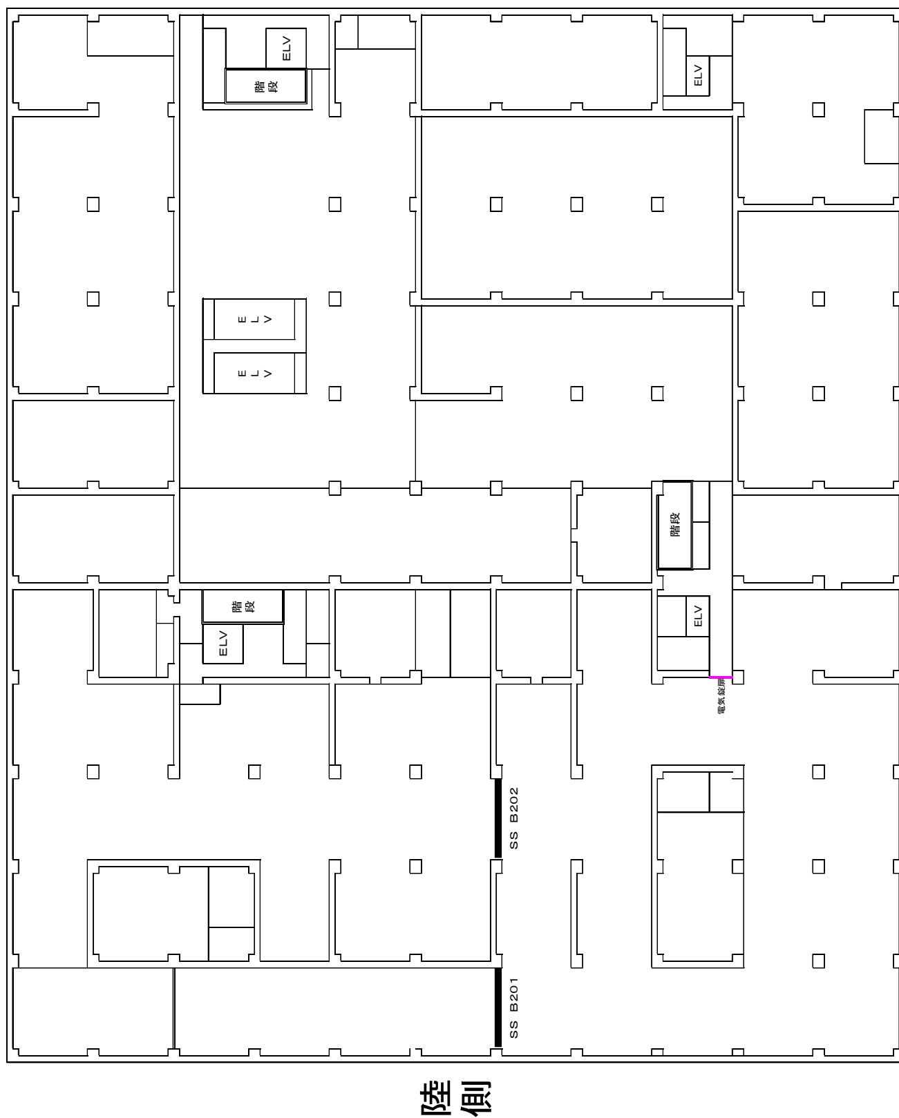
シャッター・防火シャッター配置図 (B2F)
