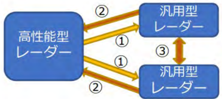
図5. 1. 1-3 高性能型レーダーと汎用型レーダーの混信の前提条件
