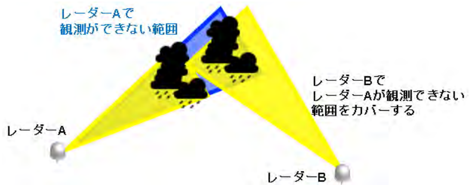
図3.5.4-2 降雨減衰時の観測の補完
