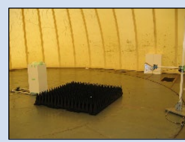
電波吸収体敷設型OATS
