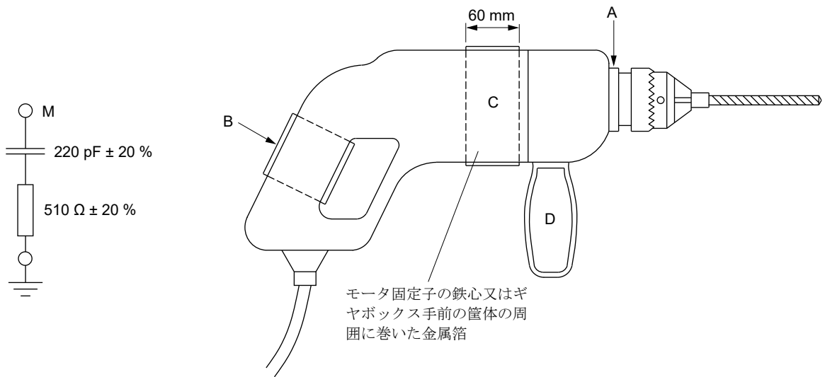
図 17 - 擬似手の RC 素子
